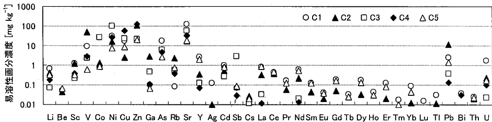
図一 6 化学工場汚泥 (C1~5) 中の易溶性画分 (交換態, 炭酸塩結合態, 鉄・マンガン酸化物結合態の合計) の濃度
