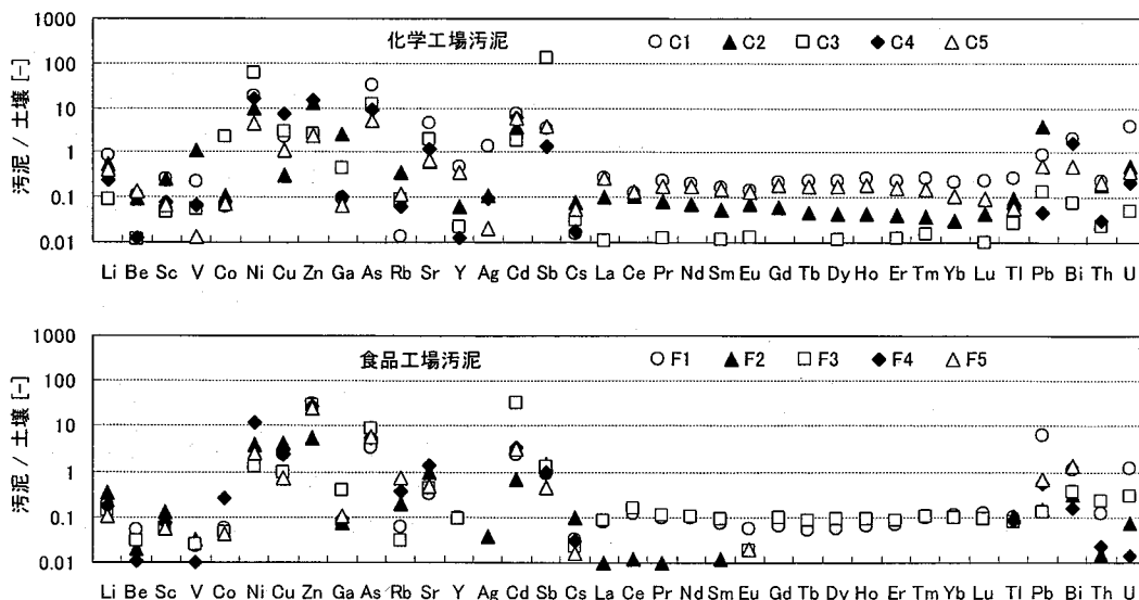
図一29(1) 廃水処理汚泥中の易溶性画分濃度の火山灰土壤中の濃度に対する割合 (化学工場汚泥, 食品工場汚泥)
