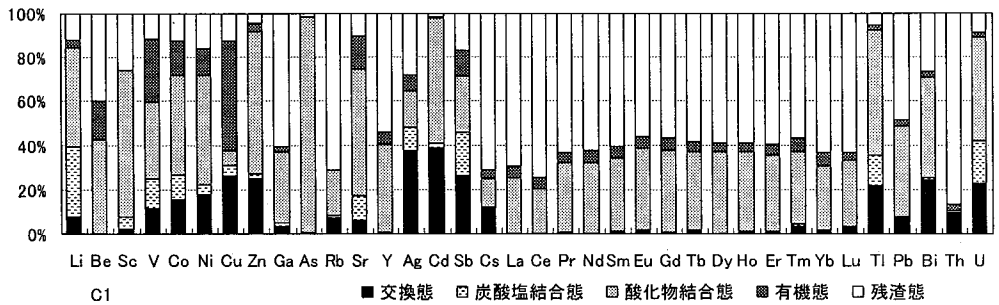
図-1 化学工場汚泥 (C1) 中の微量元素の形態別存在割合
