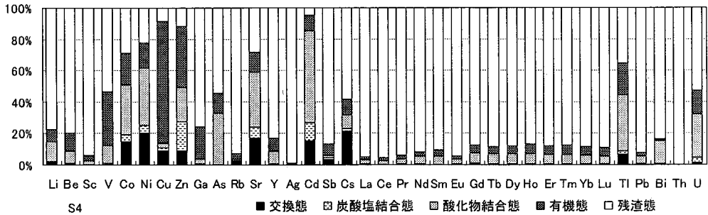
図-22 下水汚泥 (S4) 中の微量元素の形態別存在割合
