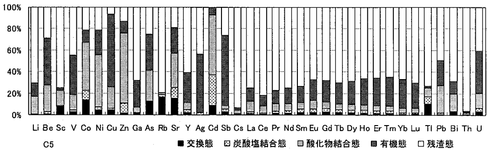
図一 5 化学工場汚泥 (C5) 中の微量元素の形態別存在割合
