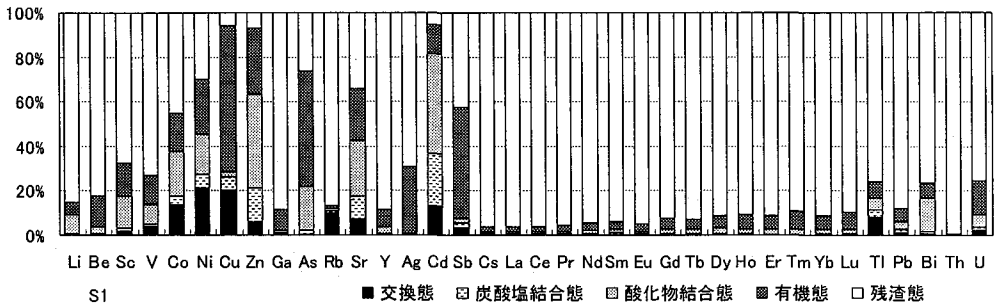
図-19 下水汚泥 (S1) 中の微量元素の形態別存在割合
