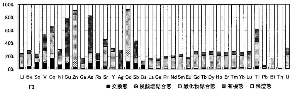
図-9 食品工場汚泥 (F3) 中の微量元素の形態別存在割合
