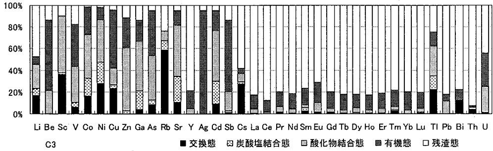
図一 3 化学工場汚泥 (C3) 中の微量元素の形態別存在割合
