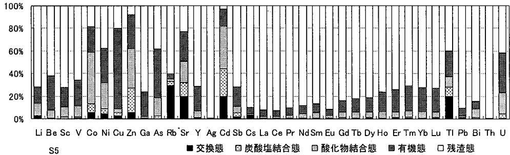
図-23 下水汚泥 (S5) 中の微量元素の形態別存在割合
