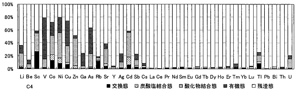
図一 4 化学工場汚泥 (C4) 中の微量元素の形態別存在割合
