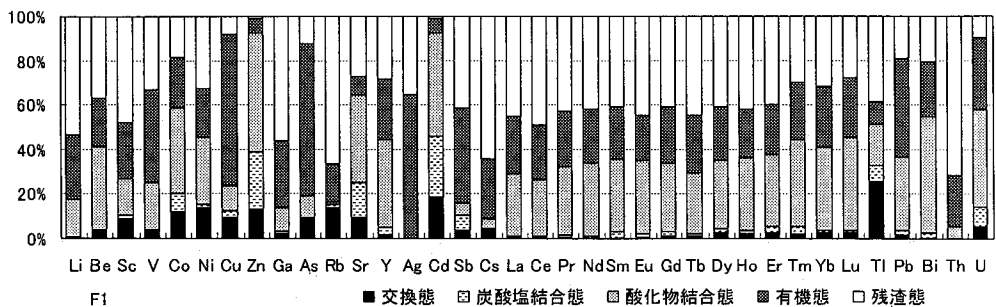
図-7 食品工場汚泥(F1)中の微量元素の形態別存在割合
