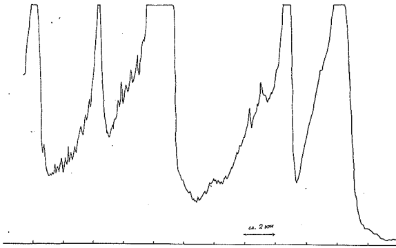
第4図 連続記録に示された赤潮の水平分布の不連続的变化
