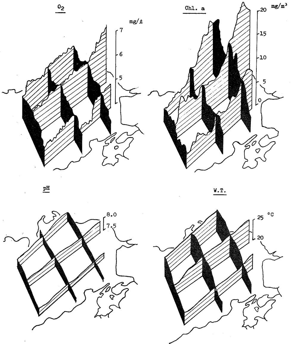
第7図 1973年6月20日、渥美湾奥部における水温、pH、溶存酸素およびクロロフィルaの連続記録結果をダイヤグラムで示したもの
