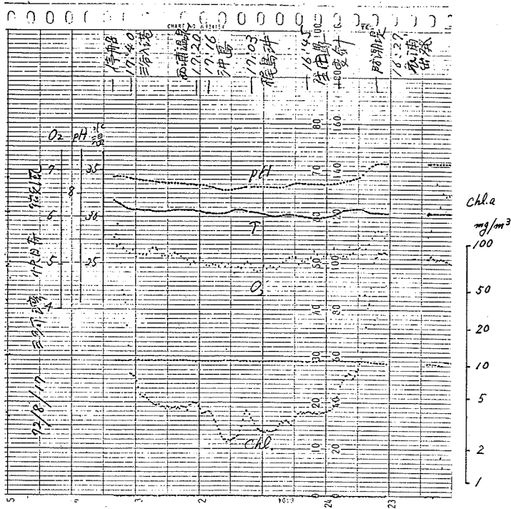
第5図 1972年8月17日、衣浦(右)から三谷(左)に至る水温、pH、溶存酸素ならびにクロロフィルの連続記録
