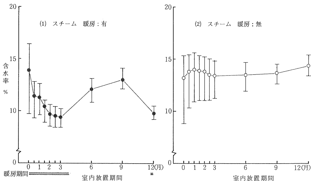
図一 3 含水率の変動
