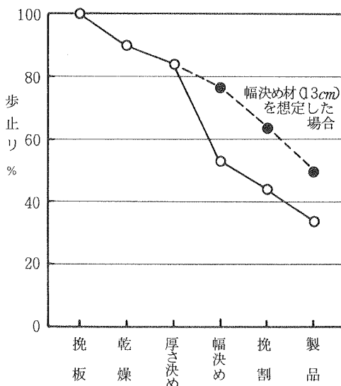
図-8 製品歩止り
