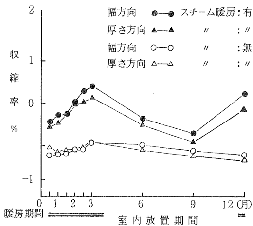
図一 4 収縮率の変動
