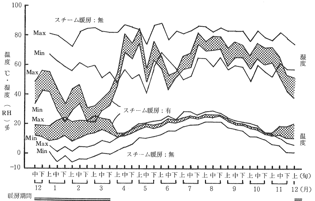
図-2 放置室内の温湿度の変動
