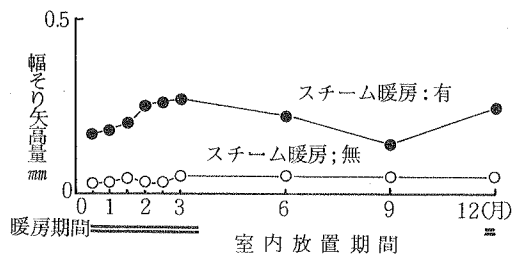
図-6 幅ぞりの変動
