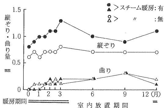
図-5 縦ぞりと曲りの変動
