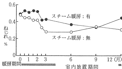
図-7 ねじれの変動
