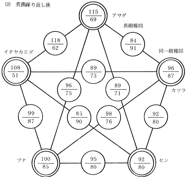
図-1 接着力と木破率
