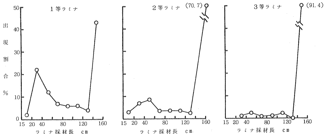
図一 9 市販 1 番玉からのラミナ採材長
