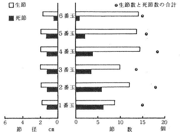
図一2 立木における地上高部位別のラミナ1枚当たりの節径と節数
