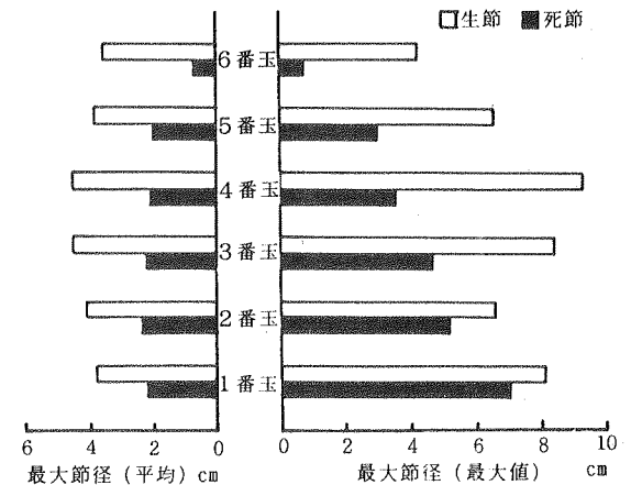
図一3 立木における地上高部位別のラミナ1枚当たりの最大節径
