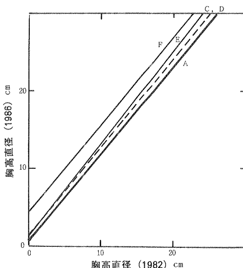
図-8 期首(1982)の胸高直径と期末(1986)の胸高直径の回帰直線
