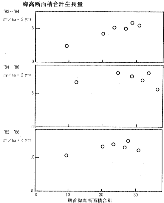
図-3 期首の胸高断面積に対する期間の胸高断面積生長量の関係
