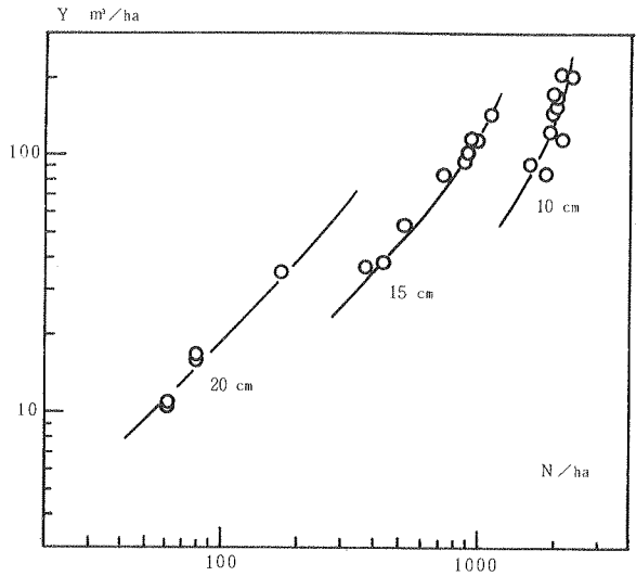
図-5 無間伐区から求めた等限界直径線
