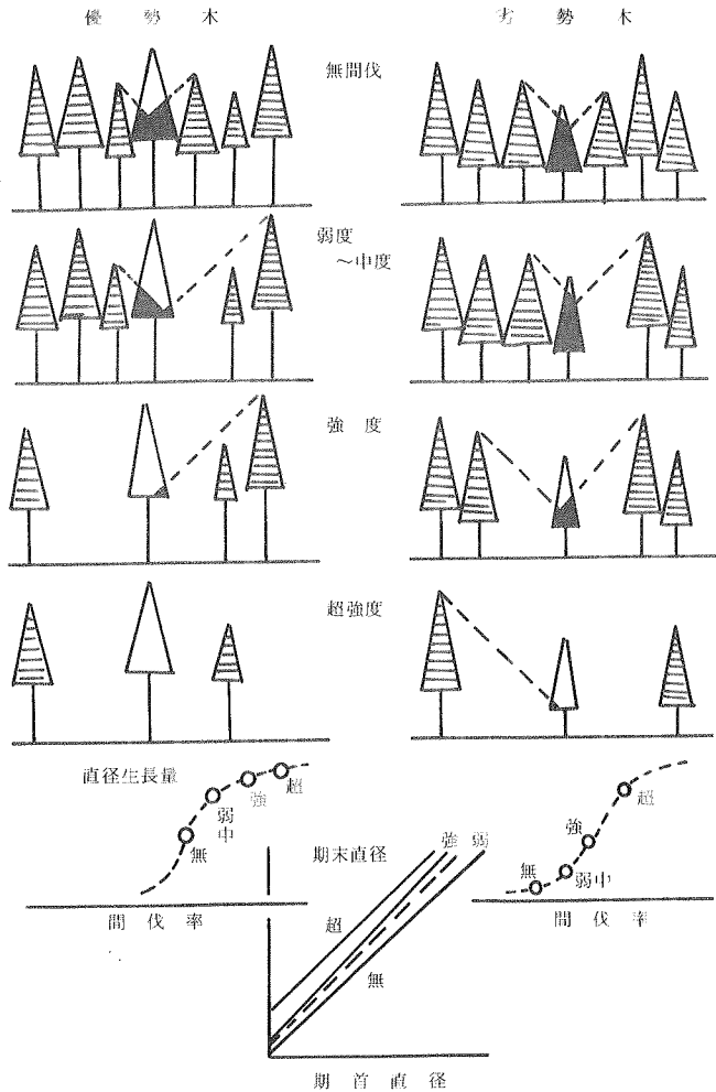
図-9 優勢木と劣勢木に対する間伐効果の模式図
