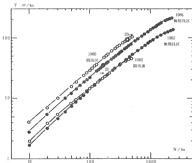
図-4 間伐前後のY-N曲線の移動 (超強度間伐区と無間伐区と比較)
