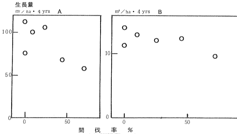
図-2 間伐率と生長量
