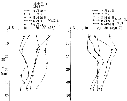
図一八 柳苗試験区における土壤溶液のNaCl換算塩濃度比C/C 1 分布（C：土壤溶液のNaCl量、C 1 ：地下水のNaCl量）
