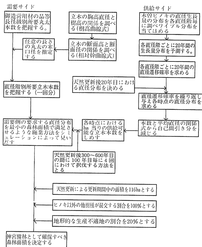
図-4 新たな視点にたって行った木曽ヒノキの保続計算の流れ図
