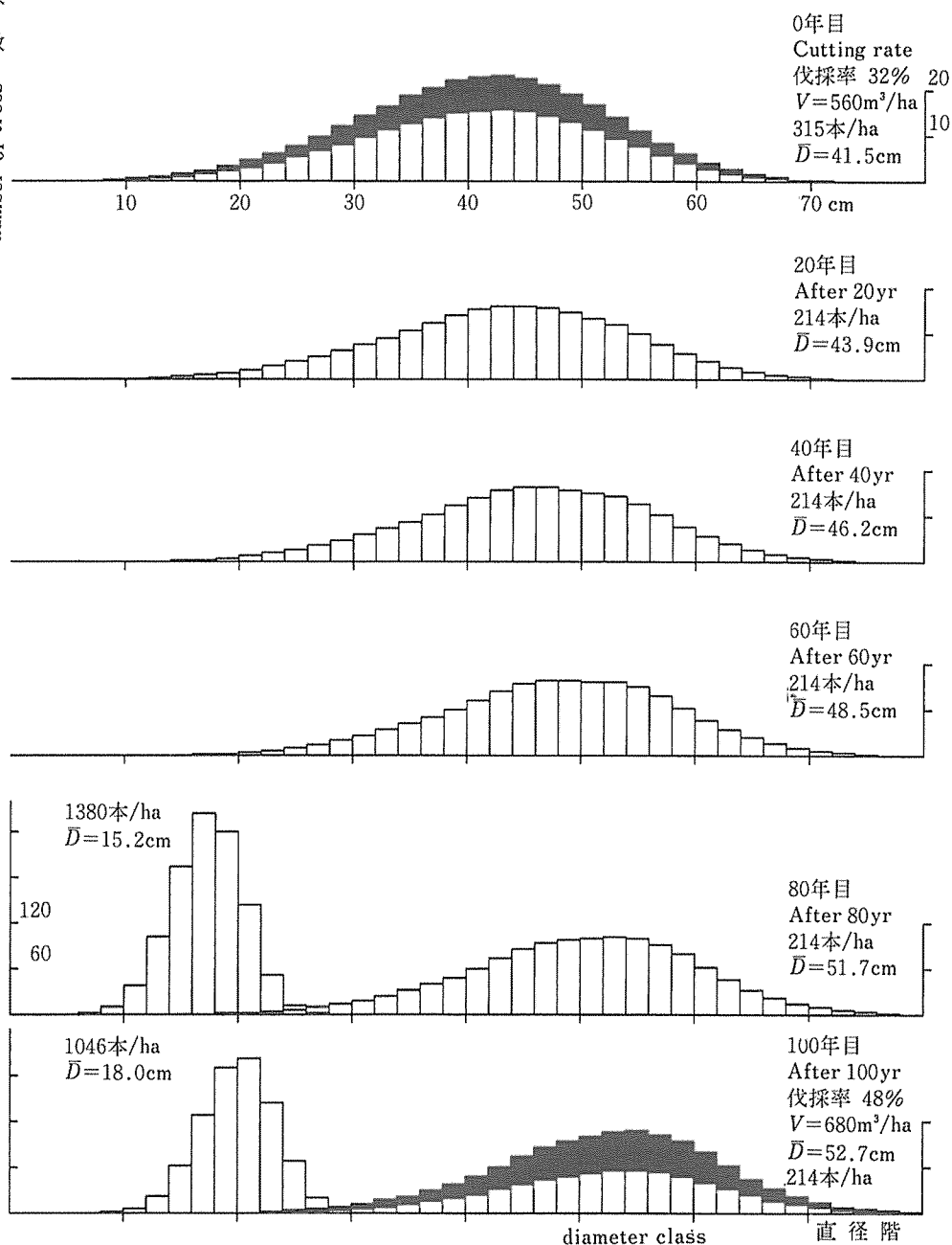
図-5 上木と下木の生長予測
