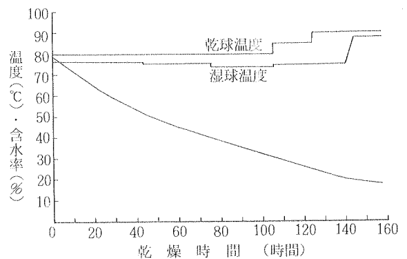
図-1 乾燥スケジュールと乾燥経過
