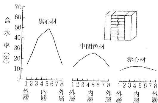
図-3 仕上り材（塗布材A）の水分分布
