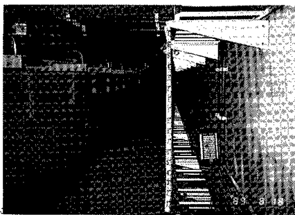
図2. 共同溝の内部
