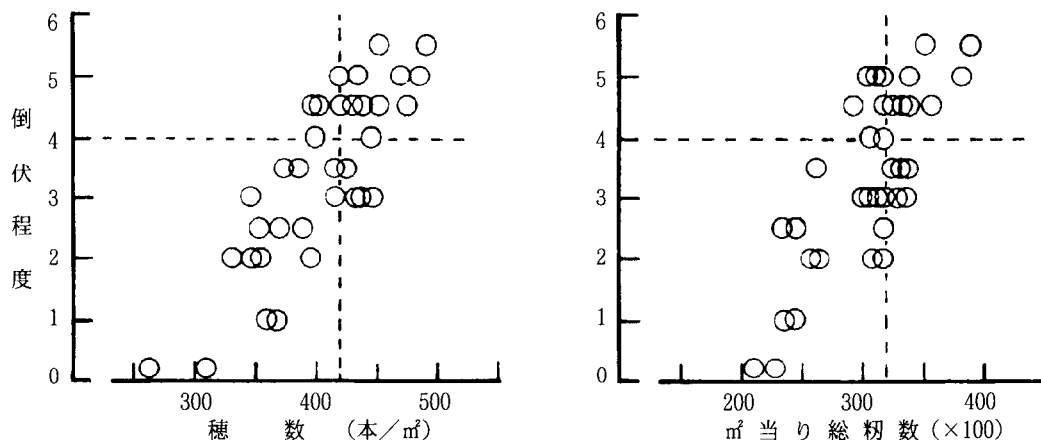
第3図 コシヒカリの穂数及び総籾数と倒伏程度の関係 (1981~1985年)
