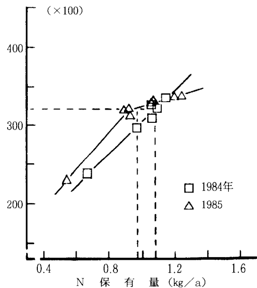
第5図 出穂期における窒素保有量と㎡当り総粒数の関係
