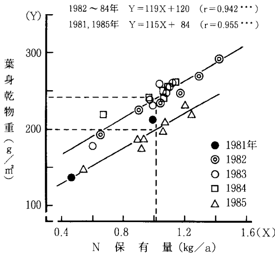
第6図 出穂期におけるコシヒカリの窒素保有量と葉身重の関係
