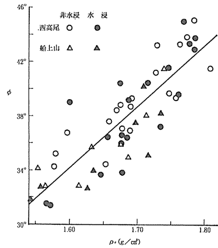
図8 凝灰岩材料の内部摩擦角 \phi と乾燥密度 \rho_d の関係
