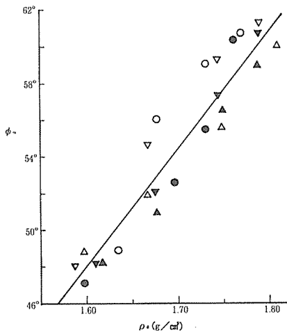
図6 砂礫材の内部摩擦角式の \phi_m と乾燥密度 \rho_d の関係
