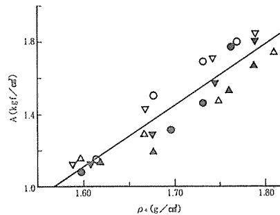
図4 砂礫材の非線形式の係数Aと乾燥密度 \rho_d の関係
