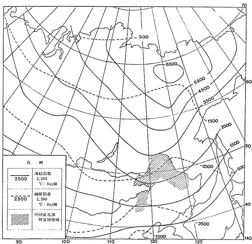
図一 1. シベリア, モンゴル, 中国東北部における凍結指数と融解指数の分布
