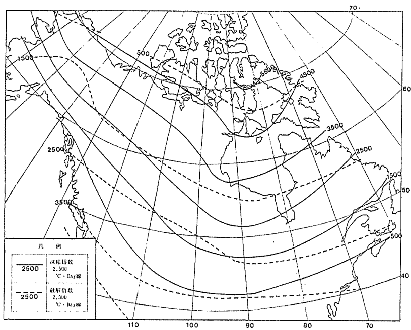
図二 2. 北アメリカ北部における凍結指数と融解指数の分布
