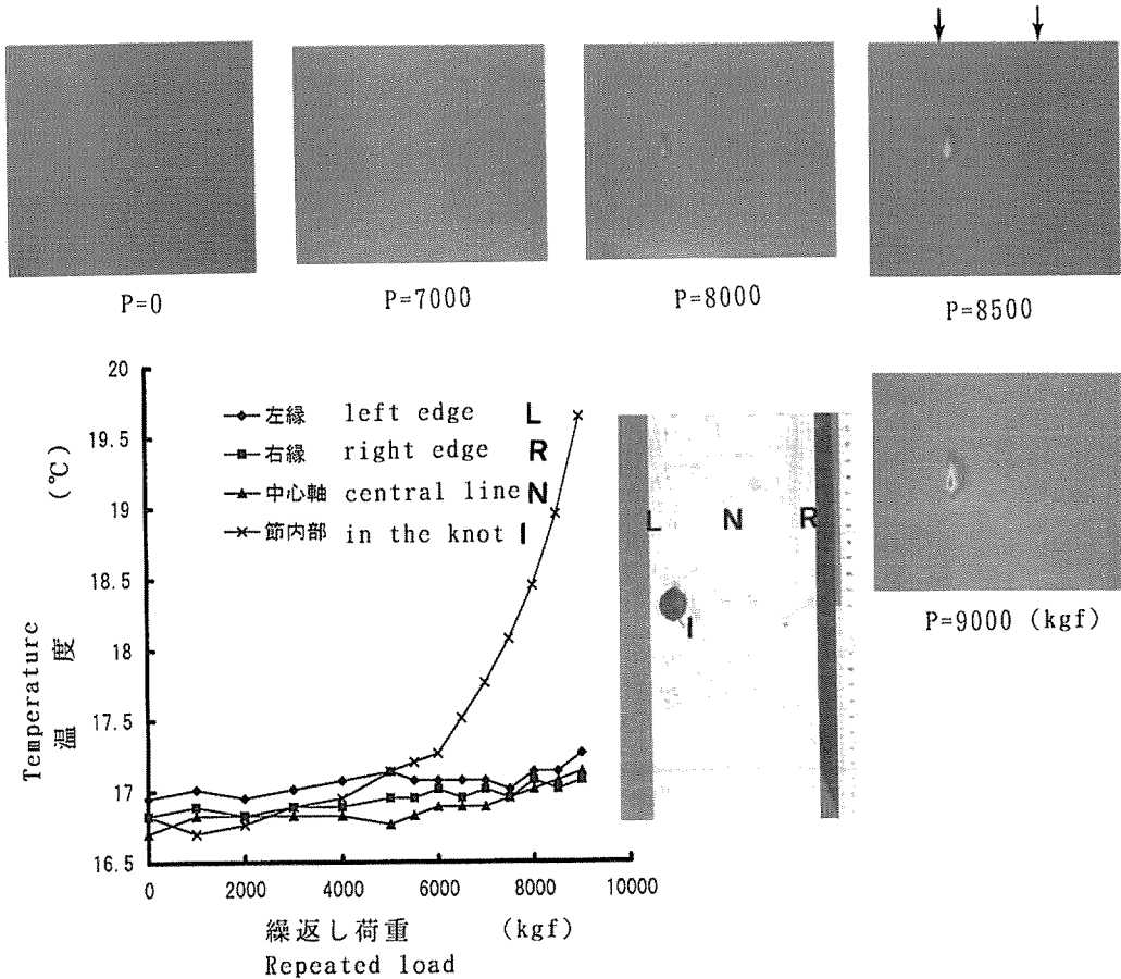
Fig. 6 繰返し縦圧縮負荷における材縁節での温度変化
