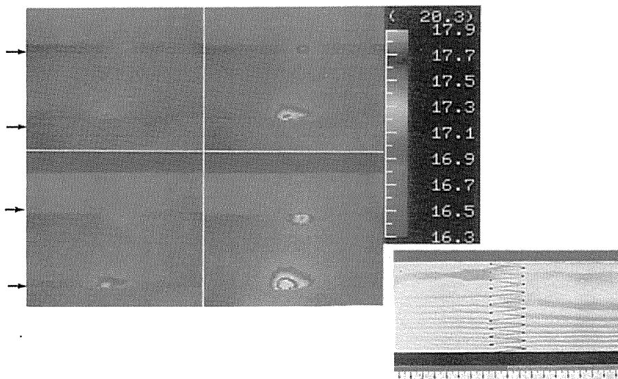
Fig. 13 繰返し曲げ負荷に伴うFJの熱画像変化 曲げ荷重 — 左上:800kgf(183kgf/cm 2 ), 左下:900kgf(206kgf/cm 2 ), 右上:1000kgf(229kgf/cm 2 ), 右下:1100kgf(251kgf/cm 2 )。括弧内の数字は外縁応力を示す。 →は材縁位置を示す。
