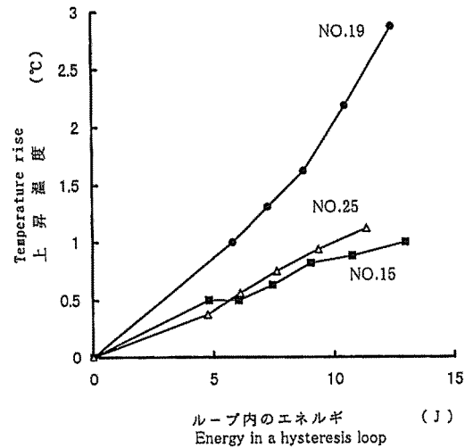
Fig. 9 荷重-変位曲線のループ内エネルギーと応力集中部の温度の関係 — 繰返し曲げ負荷, 荷重-変位曲線を静的に求めた場合 図中の数字は試験体番号を表す。No.25はFig. 3に示す試験体と同一である。
