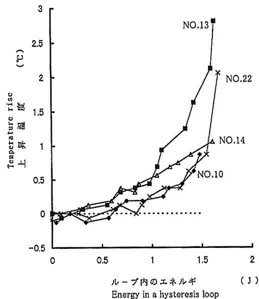
Fig. 11 各荷重レベルにおける荷重-変位曲線のループ内エネルギーと応力集中部の温度との関係 — 繰返し縦圧縮負荷の場合 — 荷重-変位曲線を繰返し負荷中に求めた場合 Fig.10 参照。
