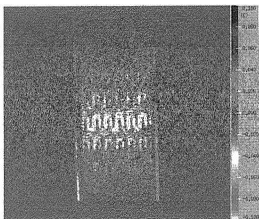
Fig. 26 熱弾性効果により求めたMCの引張荷重時と除荷時の温度差分布
