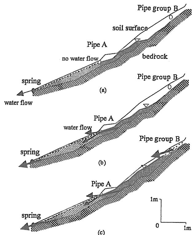
図-11. トヒノ谷の流出機構の概念図 ((a) イベント1、(b) イベント2 (c) イベント3のピーク時を示す)
