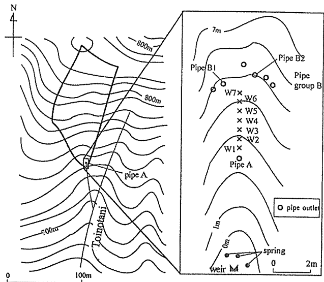
図-1. トヒノ谷の地形図および観測装置
