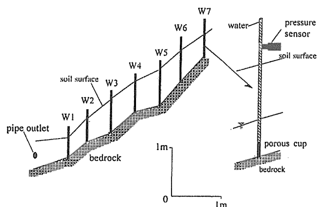
図-2. 地下水位観測点の縦断面図
