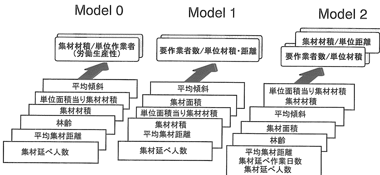
図-15 効率性改善のための最適ウェイト値に基づく入出力項目間の階層構造；間伐
