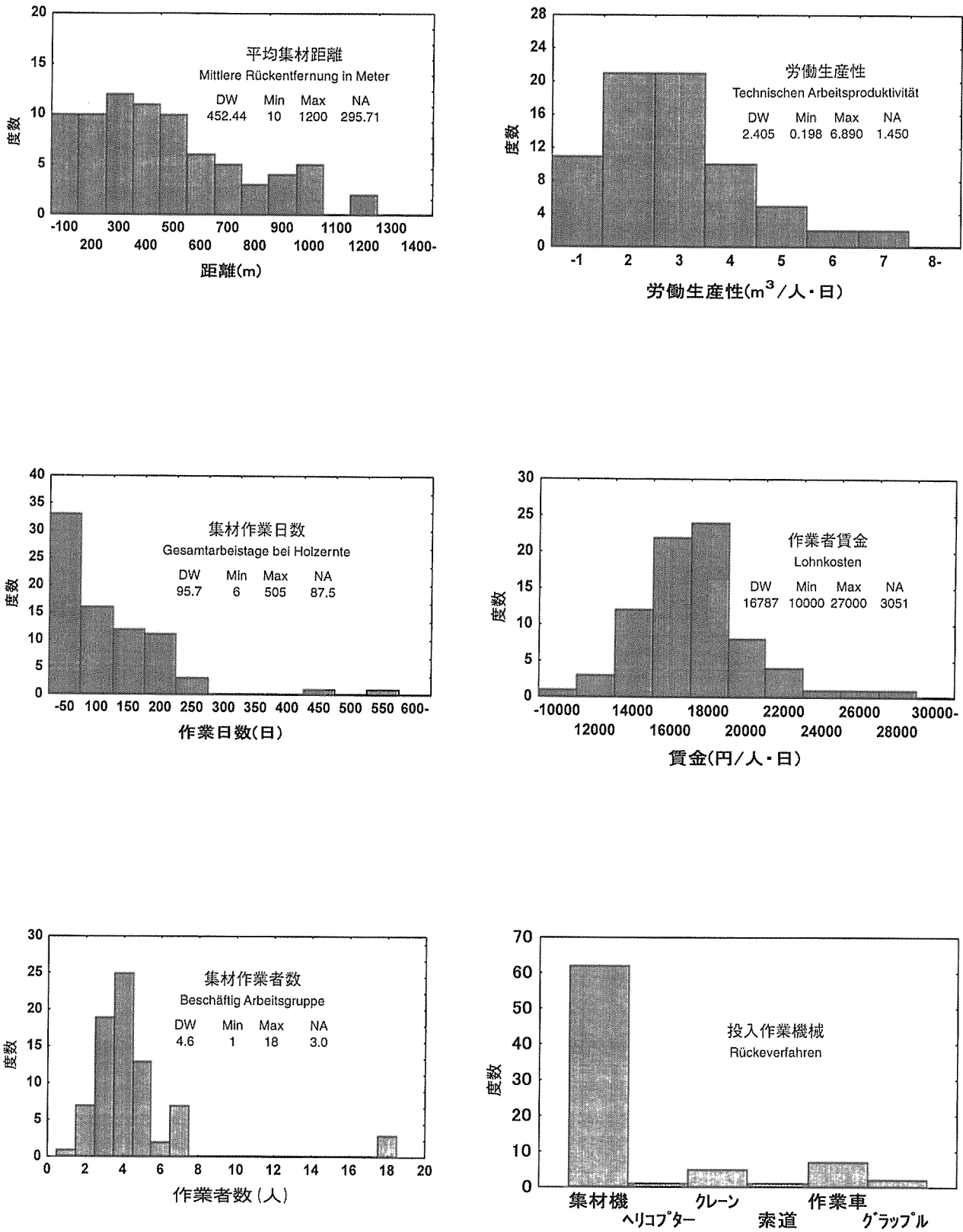
図ー 5 伐出事例単位ごとの主要項目別統計量比較；主伐 68 事例 Abb. 5 Erhebungserfolg der wichtigen Verhaltensvariablen über Produktivität, Kosten, Geländebedingungen und Arbeitskräfteinsätze bei der Holzernte in Endnutzgsbeständen mit Anzahl auswertbarer Fragebögen (68)
