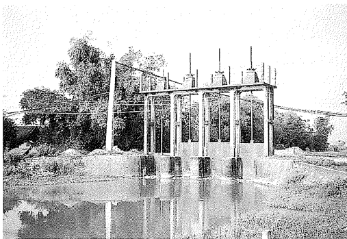
写真8 写真7の一次水路の水門 (Bac Ninh 県).
