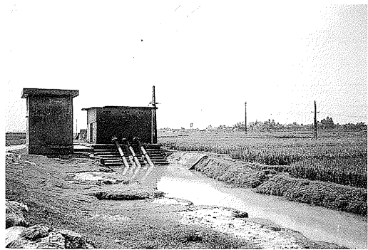
写真5 二次水路の中規模揚水機場 (Bac Ninh 県).
