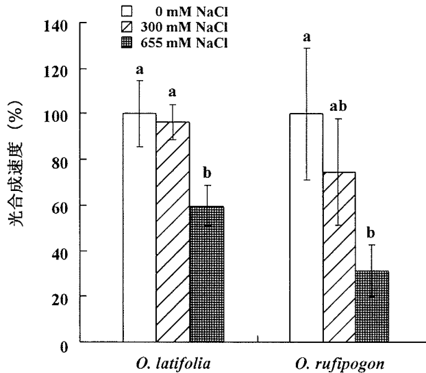
第1図 異なる NaCl 環境下での葉身光合成速度。光合成速度は酸素放出速度で評価した。0 mM NaCl 区の値を 100 とした場合の相対値で表した。 O. latifolia と O. rufipogon の 0 mM NaCl 区の値は、それぞれ 89、及び 78 \mu\text{molO}_2 \text{ mg Chl}^{-1} \text{ hr}^{-1} であった。各品種内で同一英文字のついた値間には Fisher の LSD 法により 5% 水準で有意差が無いことを示す。
