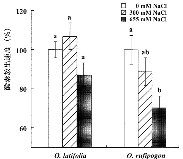
第3図 異なる NaCl 環境下でのチラコイド膜からの酸素放出速度。
