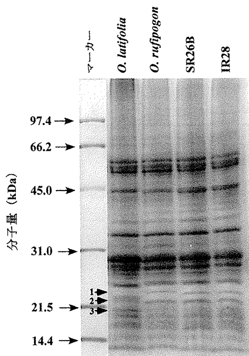
第4図 単離チラコイド膜のポリペプチド組成。
