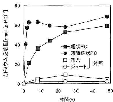
図2 PCによる土壤中カドミウム吸着量の経時的変化 ( n=2 )
