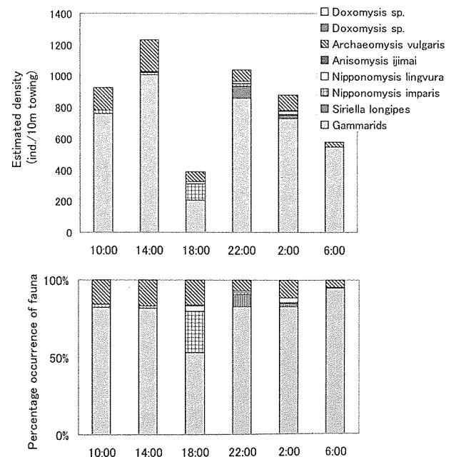
図3 長者ヶ崎海岸において採集された小型甲殻類（上段はソリネット10m曳網当たりの採集個体数、下段は組成%）
