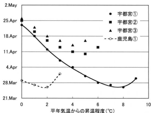
第2図 ニホンナシ‘幸水’の開花中央日に及ぼす気温上昇の影響（本條，2004）
