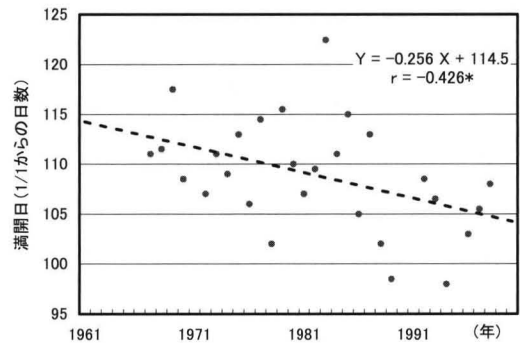
第3図 埼玉におけるニホンナシ‘幸水’開花日の推移(本條ら, 2002)
