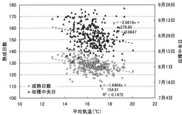
第4図 ニホンナシ‘幸水’の幼果期平均気温が果実成熟日数と収穫日に及ぼす影響(本條ら, 2005)
