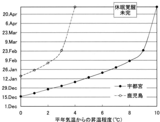
第1図 ニホンナシ‘幸水’の自発休眠覚醒時期に及ぼす気温上昇の影響（本條，2004）
