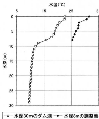
Fig.7 水温躍層形成時の水温の鉛直分布 (計測日, ダム湖: 2002年7月9日, 調整池: 2001年7月5日) Vertical profile of water temperature in summer
