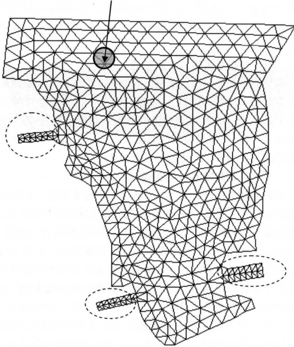
Fig.30 対象とした南椎尾調整池の有限要素分割図 (点線で囲んでいる地点は境界条件を入力するための仮想メッシュ)
