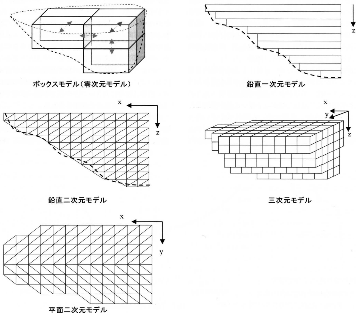
Fig.9 水質予測モデルの空間分割イメージ
