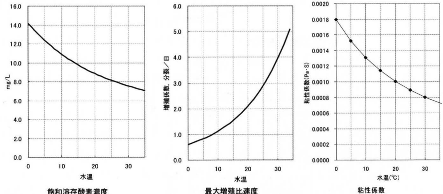
Fig.8 水温変化が水質環境に影響を与える項目 左: 水温と飽和溶存酸素濃度, 中央: 水温と藻類の最大増殖比速度, 右: 水温と密度 Relationship of water temperature and environmental factors (saturated dissolved oxygen concentration, algal growth rate, and viscosity)
