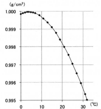
Fig.6 水温と密度
