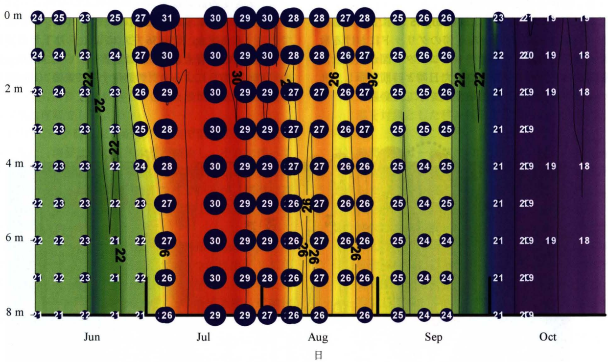
Fig.33 水温の観測値（青丸数字）と数値計算結果（コンター図）の比較 青丸の場所は観測日時と水深を、色調は温度が高（赤）から低（藍）の変化を表す。
