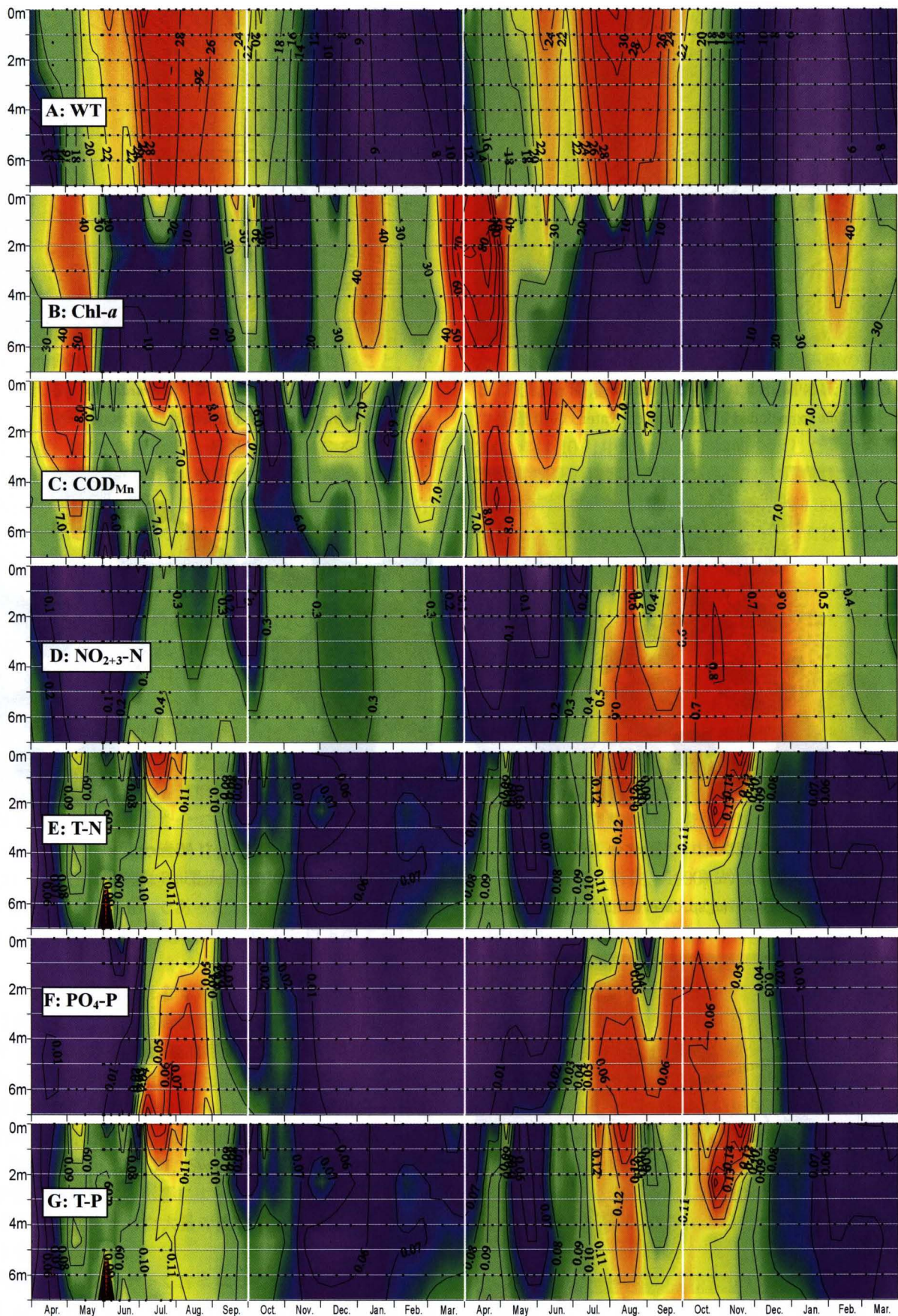
Fig.19 水質環境の季節変化。水温 (A, °C), Chl-a (B, \mu\text{g} \cdot \text{L}^{-1} ), COD Mn (C), NO 2+3 -N (D), T-N (E), PO 4 -P (F), T-P (G), C ~ G の単位は ( \text{mg} \cdot \text{L}^{-1} )。色調は濃度や温度が高 (赤) から低 (藍) の変化を表す。
