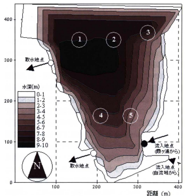
Fig.16 調整池の平面図と深浅図
