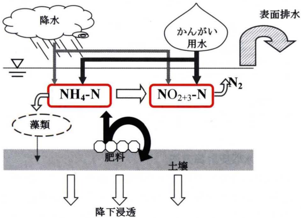
Fig.42 田面水中の溶存態窒素モデルの概念図
