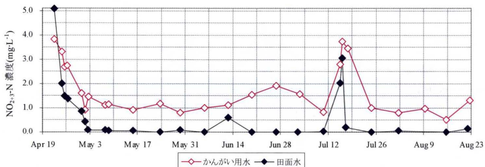
Fig.44b かんがい期間中のかんがいの用水と田面水の \text{NO}_{2+3}\text{-N} 濃度の変化
