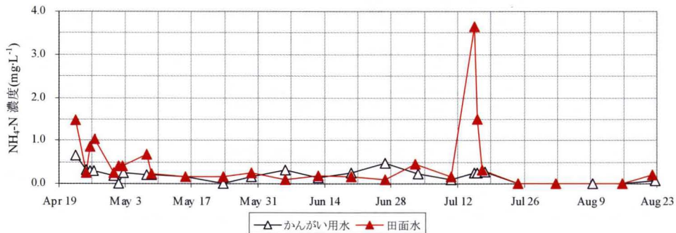
Fig.44a かんがい期間中のかんがいの用水と田面水の \text{NH}_4\text{-N} 濃度の変化
