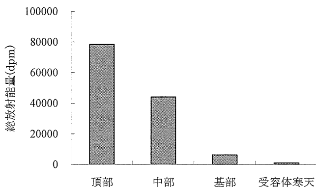
図3. 各茎切片および受容体寒天の総放射エネルギー
