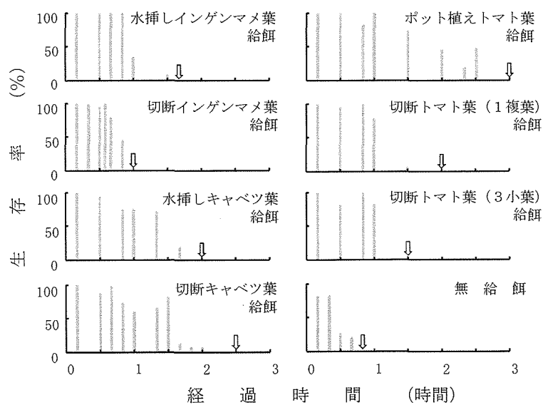
第4図 45℃条件下の各区における生存率の推移
