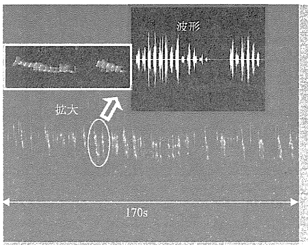
図 2. 子ラットの発した超音波の一例 上部は部分拡大のスペクトログラム及び波形
