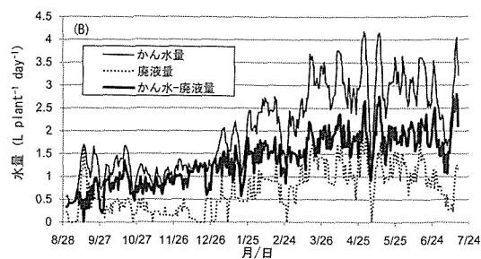
図-6 トマトの長期多段栽培期間中の細霧噴霧量 (A) かん水量および排水量 (B) の推移 グラフ (B) のデータは5日移動平均値で示した。
