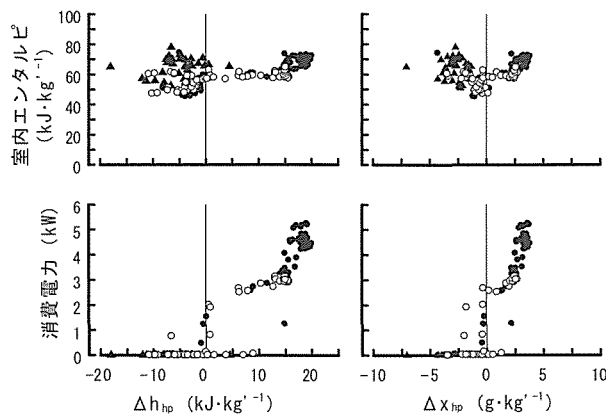
図-7 エンタルピー差 a ( \Delta h_{hp} ) および絶対湿度差 a ( \Delta x_{hp} ) と室内エンタルピーおよび消費電力との関係
