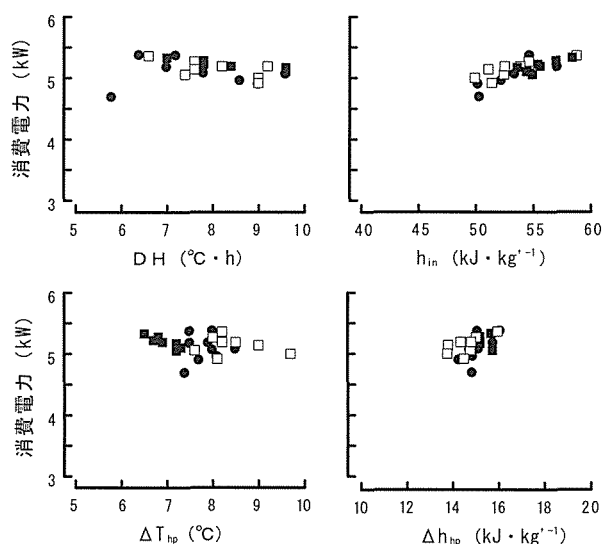
図-2 冷房デGREEアワー (DH a ), 温室内のエンタルピ (h in ), ヒートポンプ吹出口と吸込口との温度差 b ( \Delta T_{hp} ) およびエンタルピ差 b ( \Delta h_{hp} ) と消費電力との関係
