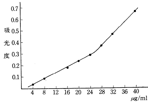
第1図 トリプシンインヒビター標準線
