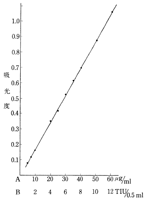
第2図 トリプシンインヒビター活性算定用 L-チロシン標準線
