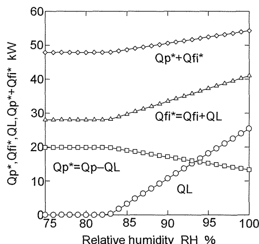
図6 除湿なしビニールハウスの温度に関する予測計算例
