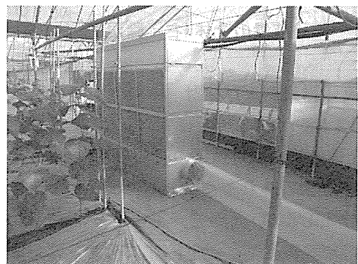
図 1 温室内に設置・稼働中の除湿ユニット
