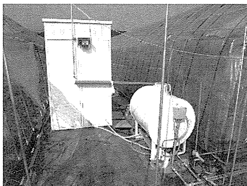
図2 温室外に設置した再生ユニット
