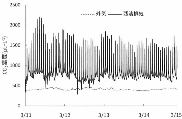
図－4 残渣から排出されるガス中の \text{CO}_2 濃度 (測定日：3月11日～15日)
