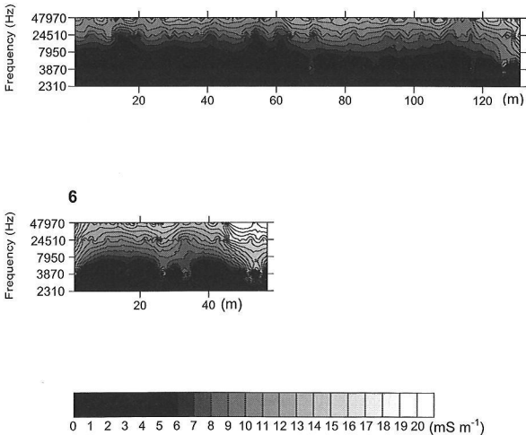
Fig. 4 間伐の違いによる見かけの電気伝導度の鉛直分布の違い. No. 13 間伐された土地, No.6 間伐遅れが見られる土地. Vertical profiles of electric conductivity differed by thinning. No. 13 The thinning site, No. 6 The delayed thinning site.
