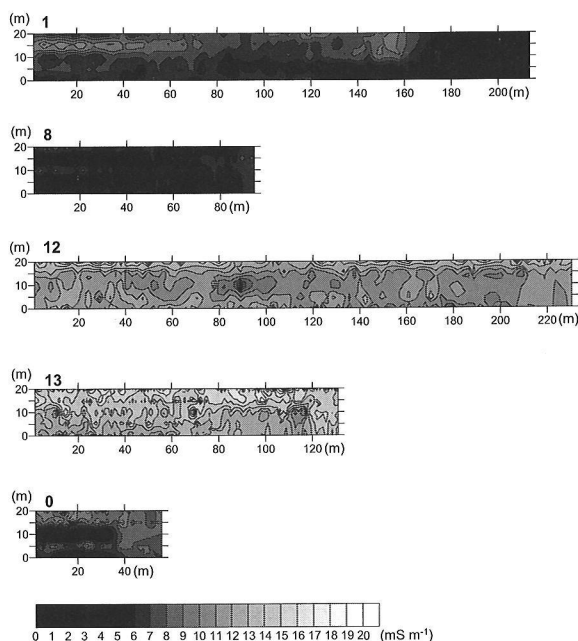
Fig. 6 間伐の行われているサイトの見かけの電気伝導度の水平分布 (周波数 47973 Hz).
