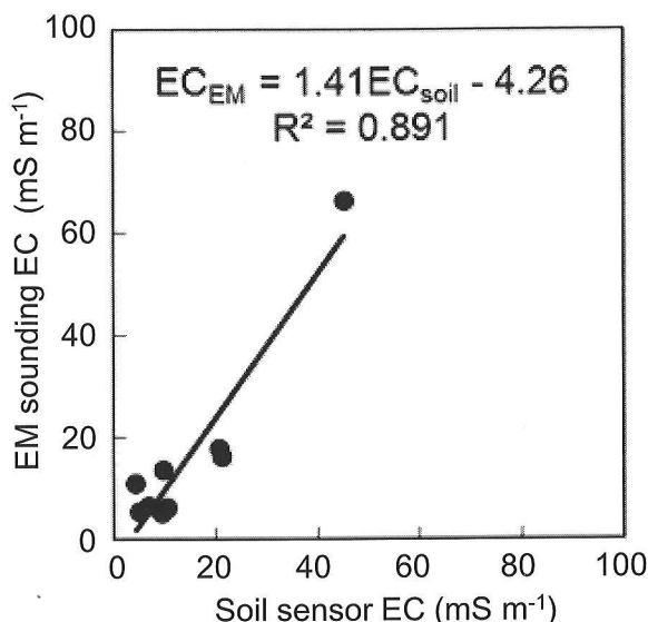
Fig. 5 電磁探査と土壌センサーの見かけの電気伝導度の比較.
