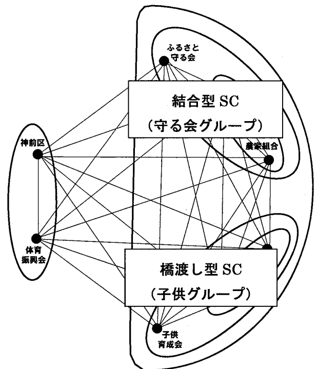
図4 SN構造とSC指標との関係イメージ
