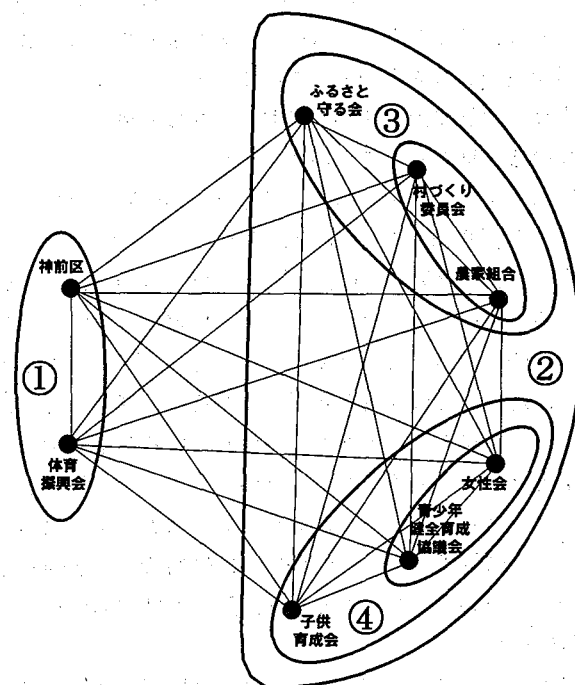
図 2 守る会の SN 構造の階層性
