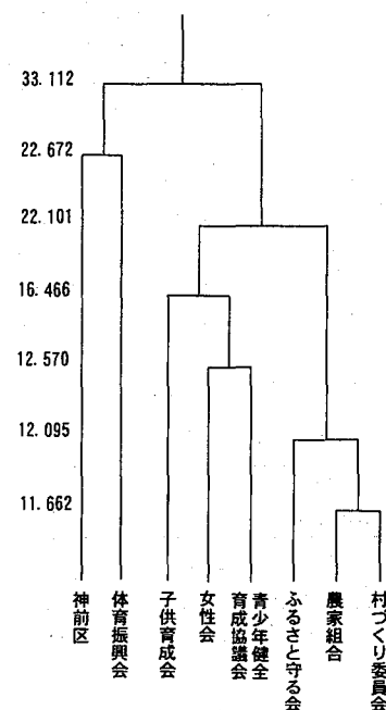
図 1 デンドログラム
