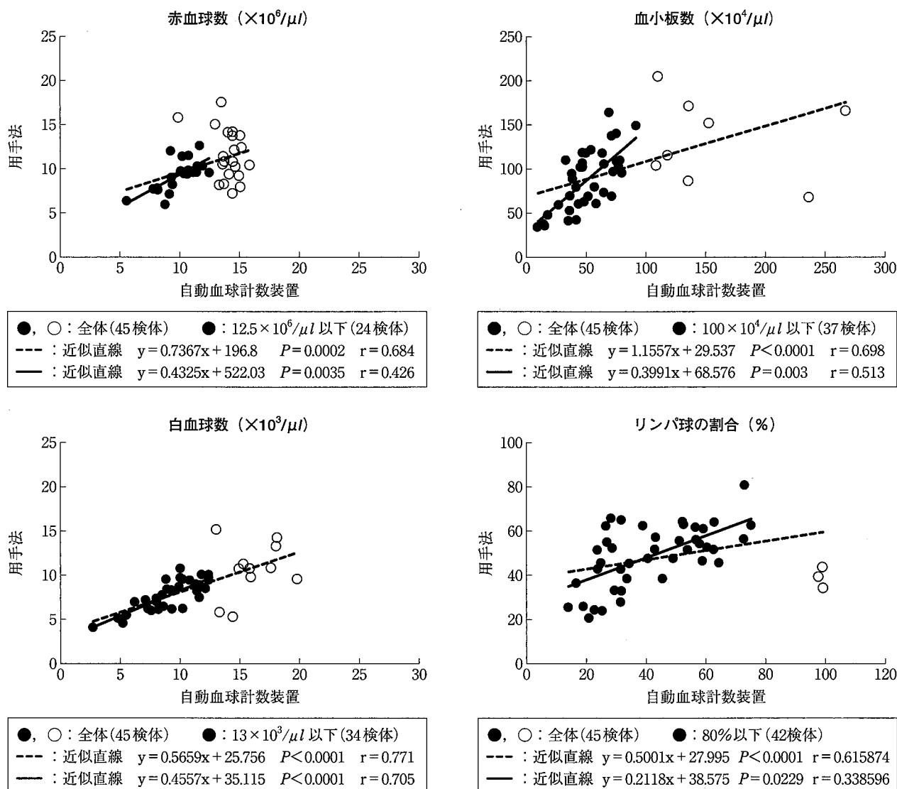
図 用手法と自動血球計数装置間での黒毛和種子牛の赤血球数, 血小板数, 白血球数及びリンパ球の割合の相関
