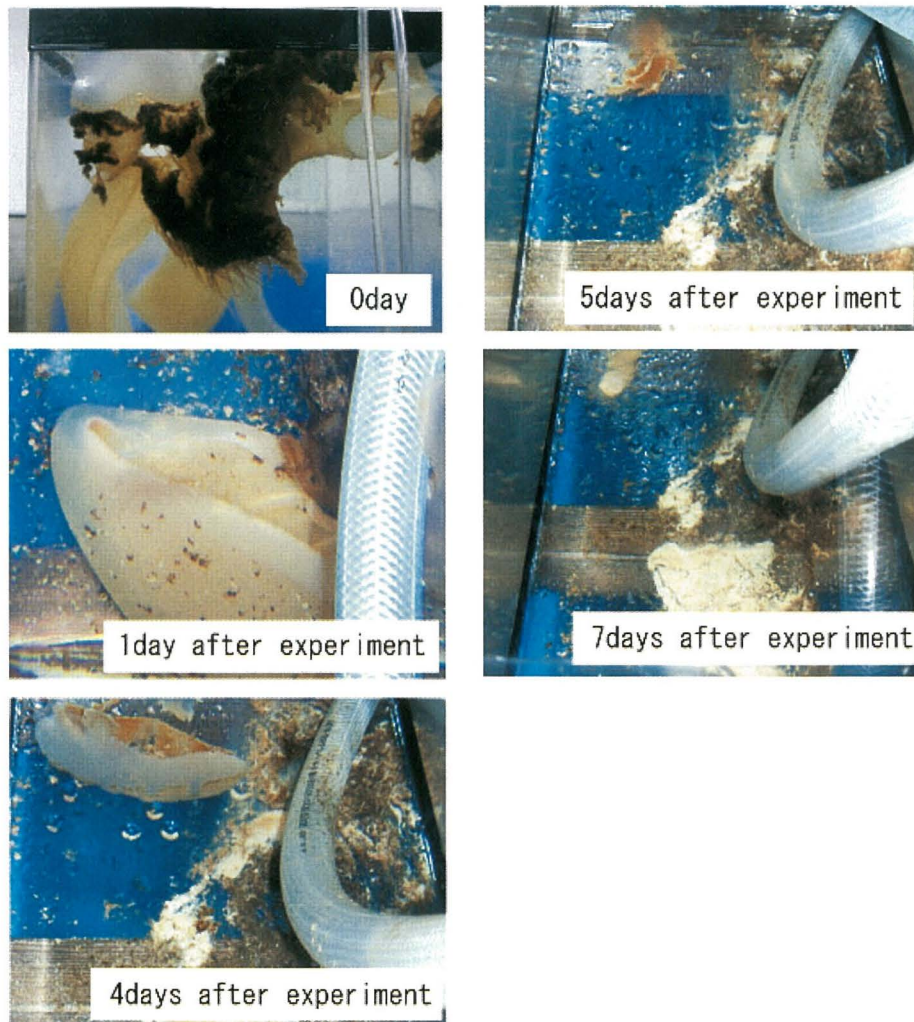
Fig. 2 A decomposition process of N. nomurai in surface sea water 表層海水中におけるエチゼンクラゲの分解過程
