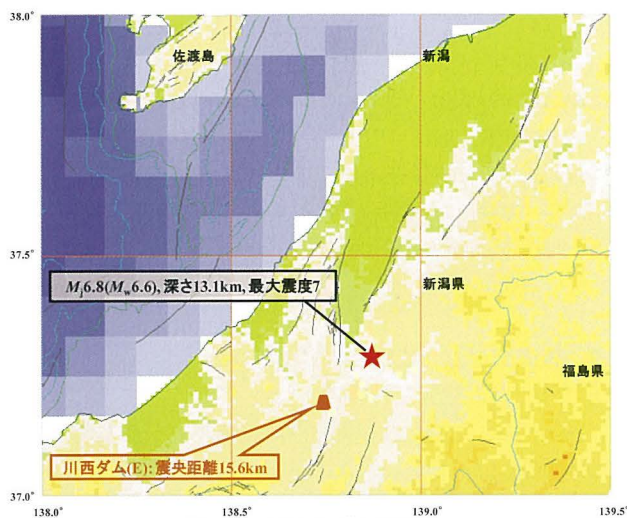
Fig. 16 震央とダム位置 Epicenter and dam position
