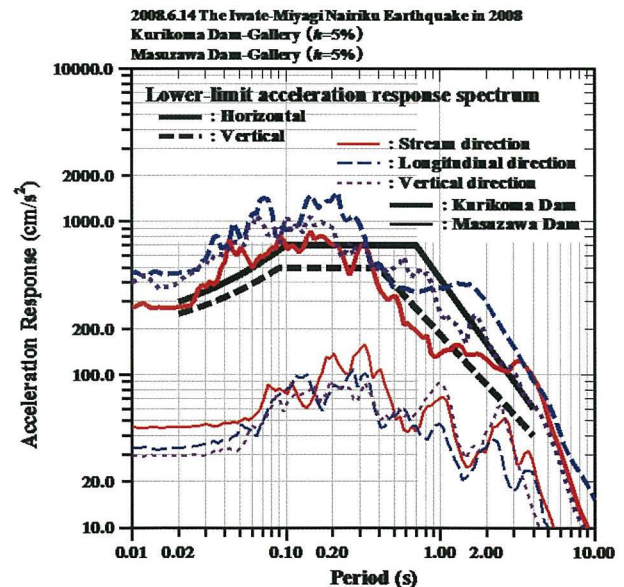
Fig. 35 加速度応答スペクトル (栗駒ダムの基部監査廊と柘沢ダムの河床部監査廊) Acceleration response spectrum (Gallery of Kurikoma Dam and Masuzawa Dam)
