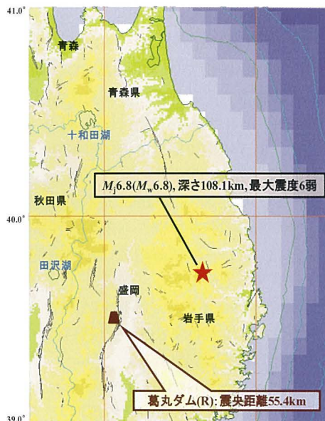
Fig. 39 震央とダム位置 Epicenter and dam position
