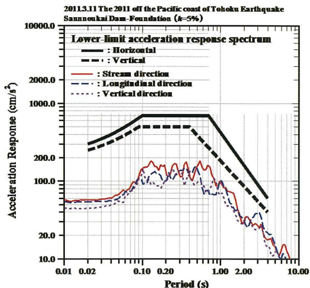
Fig. 49 加速度応答スペクトル（河床部監査廊） Acceleration response spectrum (Foundation)
