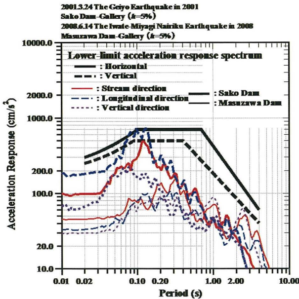
Fig. 36 加速度応答スペクトル (佐古ダムと枧沢ダムの河床部監査廊) Acceleration response spectrum (Gallery of Sako Dam and Masuzawa Dam)
