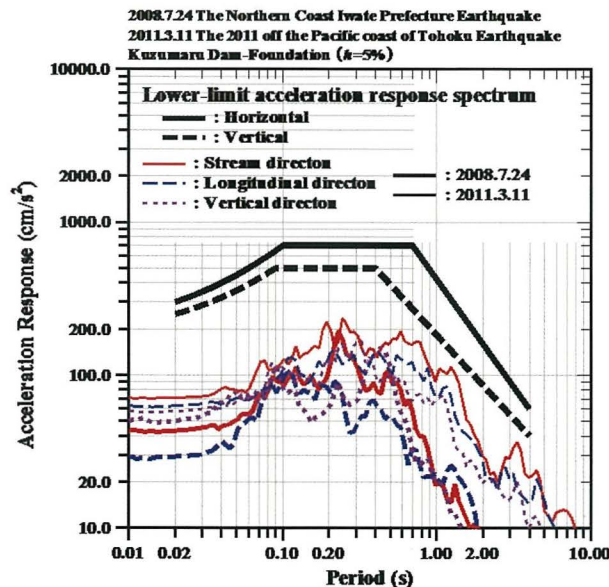
Fig. 51 「岩手県沿岸北部の地震」(河床部監査廊)と「平成23年(2011年)東北地方太平洋沖地震」の加速度応答スペクトル (河床部監査廊) Acceleration response spectrum (Foundation) at “The Northern Coast Iwate Prefecture” and “The 2011 off the Pacific coast of Tohoku Earthquake”
