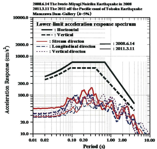
Fig. 65 「平成20年(2008年)岩手・宮城内陸地震」(河床部監査廊)と「平成23年(2011年)東北地方太平洋沖地震」の加速度応答スペクトル (河床部監査廊) Acceleration response spectrum (Gallery) at “The Iwate-Miyagi Nairiku Earthquake in 2008” and “The 2011 off the Pacific coast of Tohoku Earthquake”
