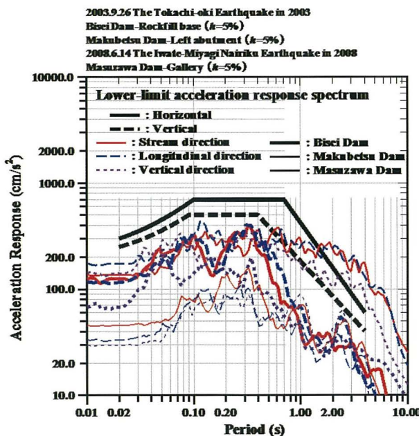
Fig. 37 加速度応答スペクトル (美生ダムのコンクリート部分河床部監査廊と幕別ダムの左岸地山と枧沢ダムの河床部監査廊) Acceleration response spectrum (Gallery of gravity at Bisei Dam, left abutment of Makubetsu Dam and gallery of Masuzawa Dam)
