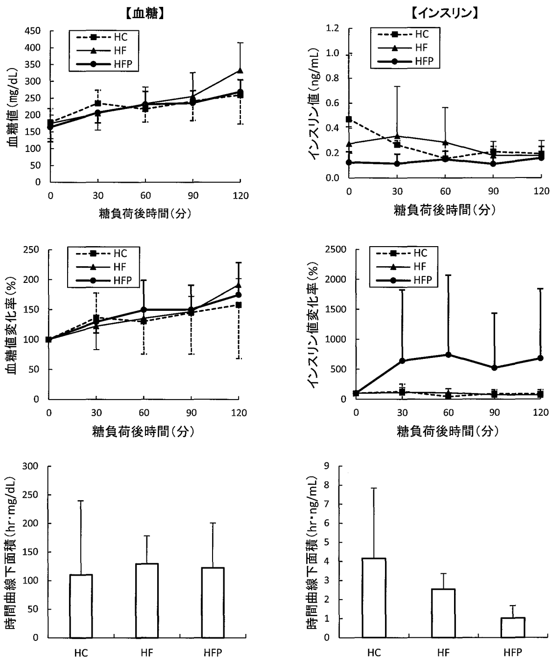
図1 経口糖負荷試験における血糖値とインスリン値の経時変動(6ヶ月後) データを平均値±SDで示す。HC, 高炭水化物食群 (n=3): HF, 高脂肪食群 (n=4): HFP, 高脂肪食+D-キシコース群 (n=4).
