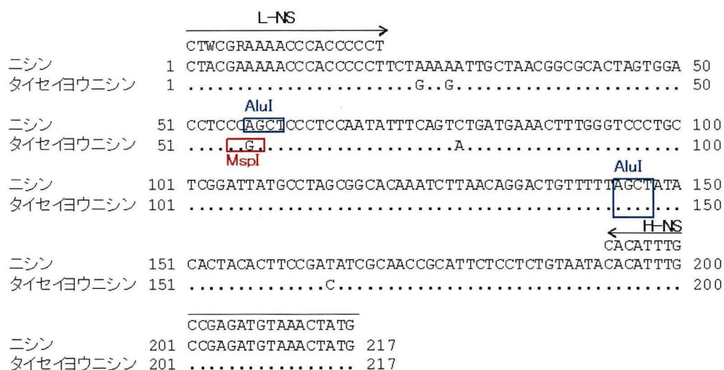
図 1 ニシンとタイセイヨウニシンの Cytb 遺伝子領域の部分配列
