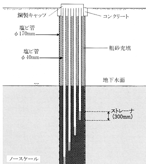
Fig.5 ババウ島地下水観測孔構造図（Fry and Falkland, 2011に 加筆）
