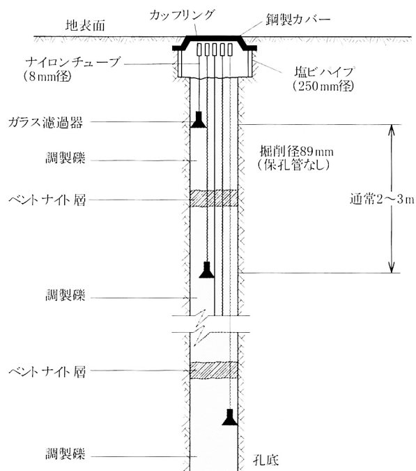
Fig.7 リフカ島地下水観測孔構造図（Woodroffe and Falkland, 1997）
