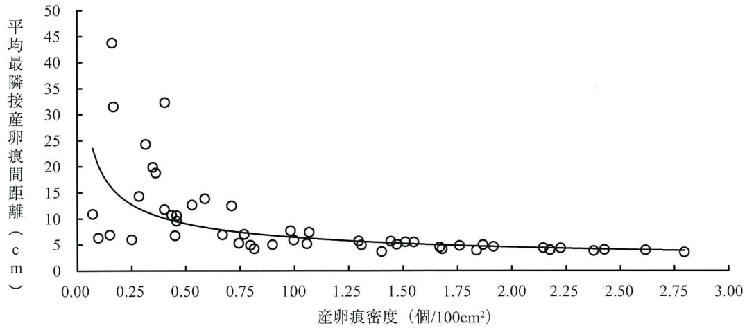
図-2 2008年度枯死木における産卵密度と平均最隣接産卵痕間距離の関係
