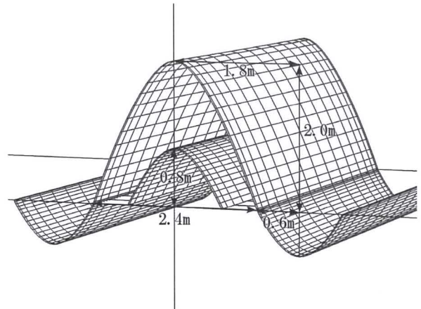
図- 5 土塁の模式図 図中の外側が構築時の形状、内側が現在の形状を示す。
