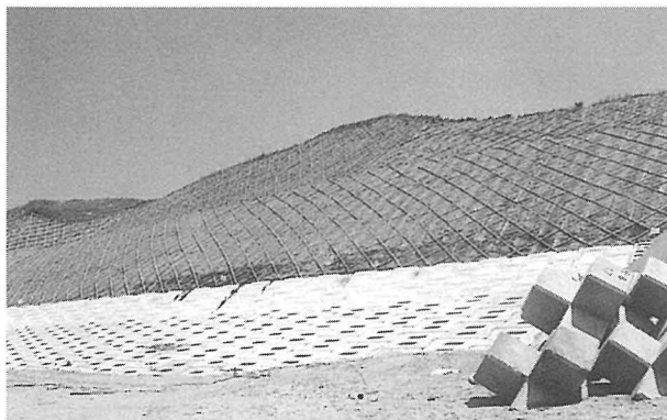
写真3 緩傾斜堤（1997年〈平成9年〉）
