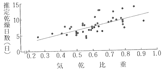
図-1 比重と推定乾燥日数の関係
