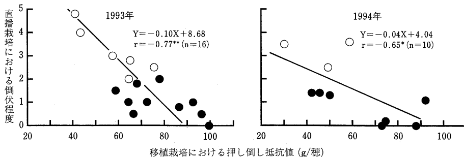
第3図 移植栽培での押し倒し抵抗値と直播栽培での倒伏程度との関係。図中の記号は第1図を参照。*, **は各々信頼水準 95, 99% で有意。
