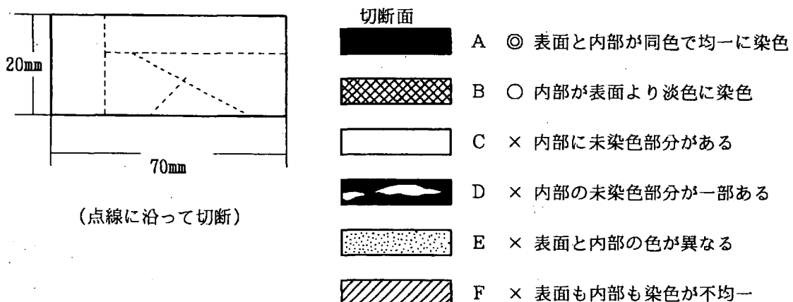
図1-1 染色木材の切断方法と浸透性の判定基準
