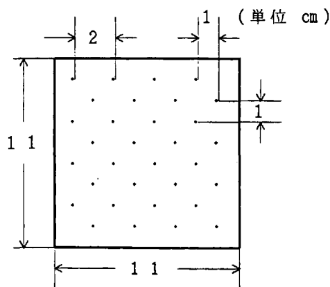
図4-1 試片の孔パターン
