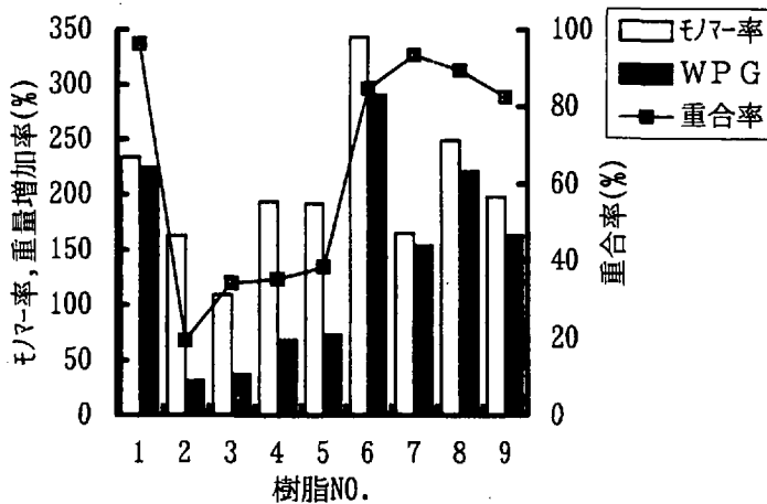
図2-1 樹脂液別の注入性
