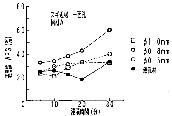
図4-4 MMA の浸透性
