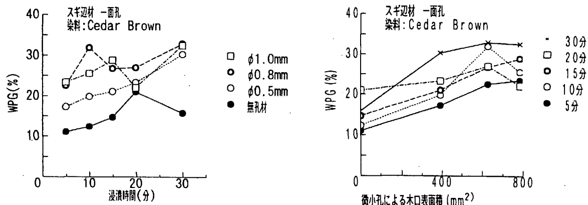
図4-2 Cedar Brown の浸透性
