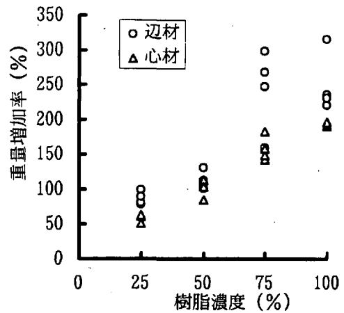
図2-2 樹脂濃度とWPG (No.1 : NKエステル)
