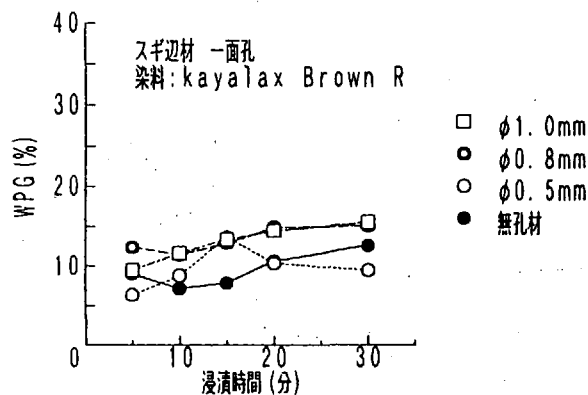
図-3 Kayalax Brown R の浸透性
