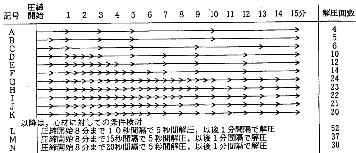
図3-1 圧縮サイクル
