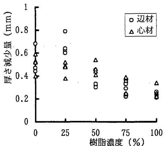
図2-5 摩耗による厚さ減少 (No.1 : NKエステル)
