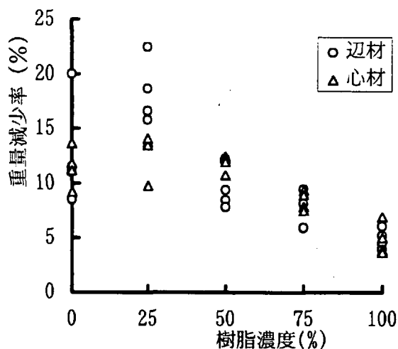
図2-4 摩耗による重量減少 (No.1 : NKエステル)
