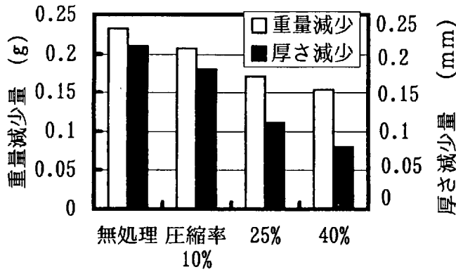
図3-2 圧密材の摩耗性
