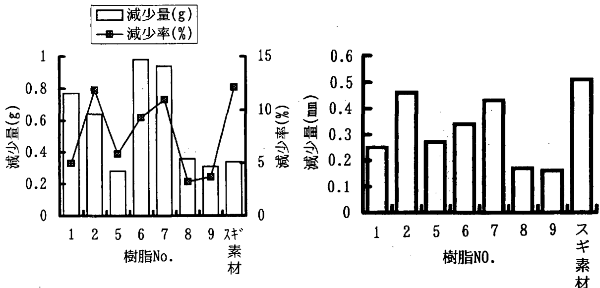
図2-3 樹脂液別の摩耗性
