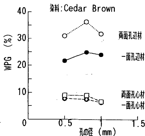
図4-5 両面孔の効果
