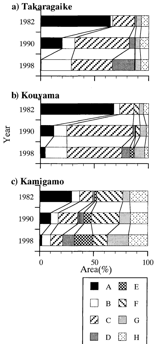
図-3 宝ヶ池, 神山, 上賀茂の各地域における各林分タイプの面積の推移。
