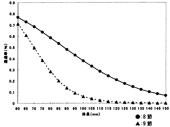
図10 角目網による通過率（本田、1990による）
