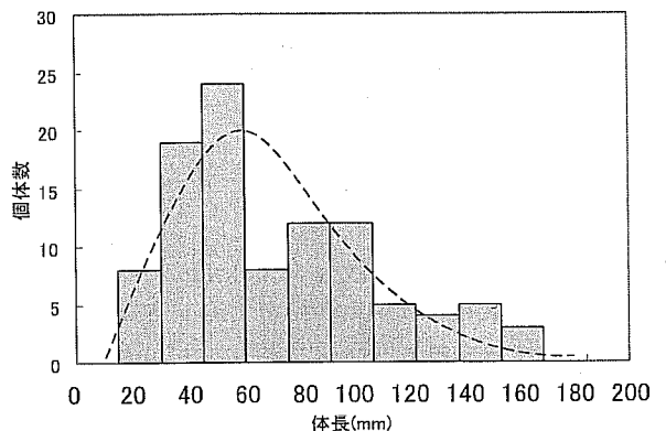
図3 飼育個体頻度分布へのゴンベルツ曲線の当てはめ
