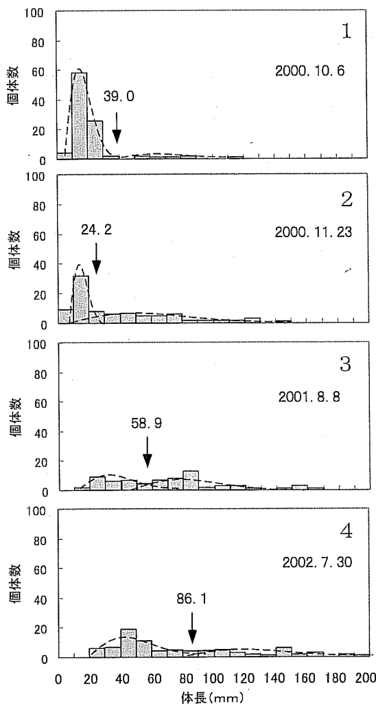
図9 調査日別サイズ別小型群の体調組成 (破線はゴンベルツ曲線, ↓で放流個体と天然個体を区分)
