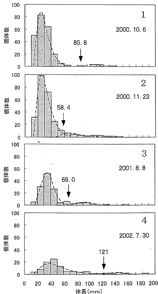
図6 調査日別サイズ別大型群の体組成 (破線はゴンペルツ曲線, ↓で放流個体と天然個体を区分)
