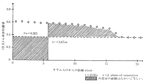
第1図 多腐植質黒ボク土カラムへの0.1M CaCl 2 溶液の浸潤過程における水分分布
