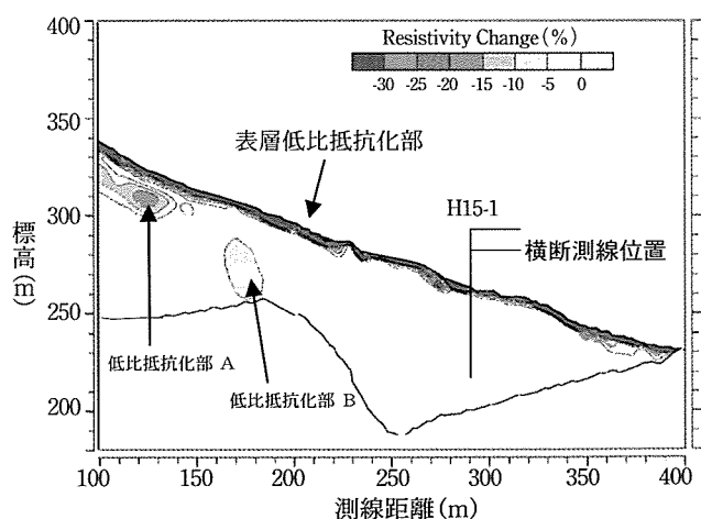
Fig. 4 縦断測線における比抵抗断面図(2004.2)
