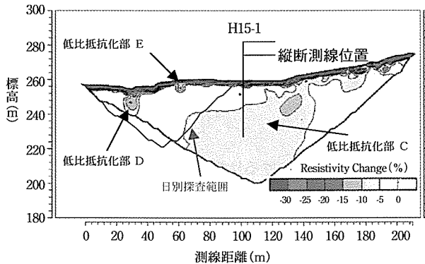
Fig. 6 2004.2をバックグラウンドとした2004.9の比抵抗変化率分布
