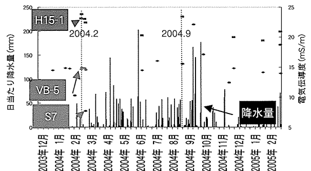
Fig. 9 調査孔(H15-1,VB-5,S7)における電気伝導度の変化
