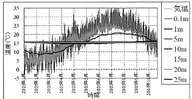
Fig. 7 調査孔H15-1における深度別地中温度変化
