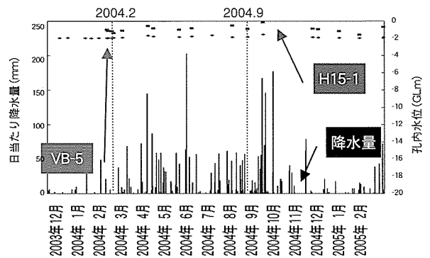
Fig. 8 調査孔(H15-1,VB-5)における地下水位の変化
