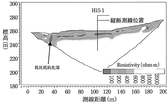
Fig. 5 横測線における比抵抗断面図(2004.2)
