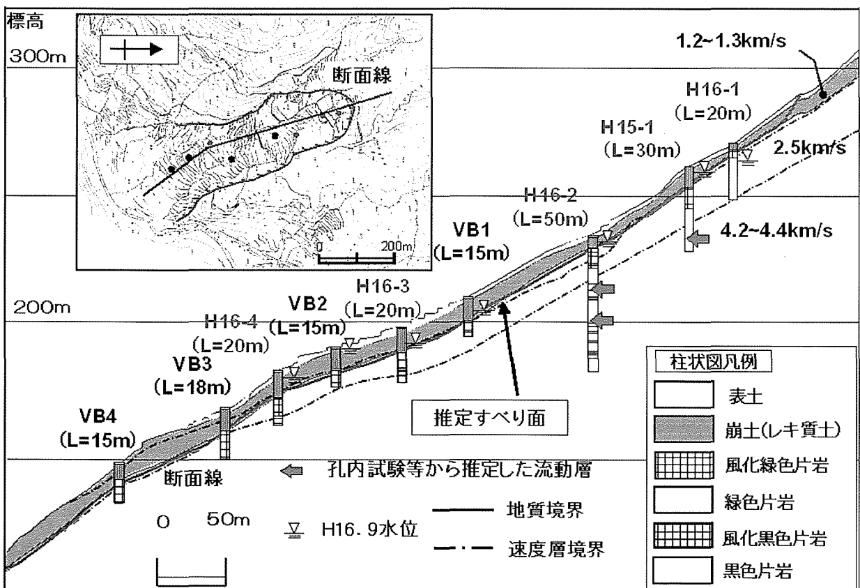
Fig. 2 試験地地すべり地質断面図
