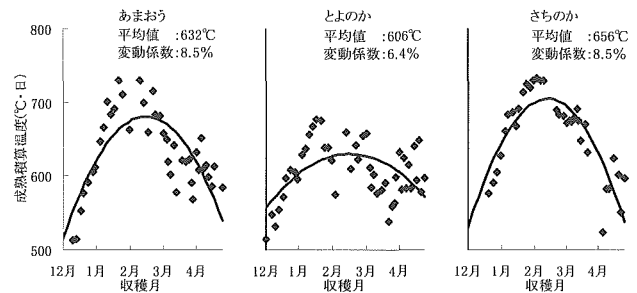
第2図 ‘あまおう’ ‘とよのか’ および ‘さちのか’ における収穫時期と成熟積算温度 (2004年度)
