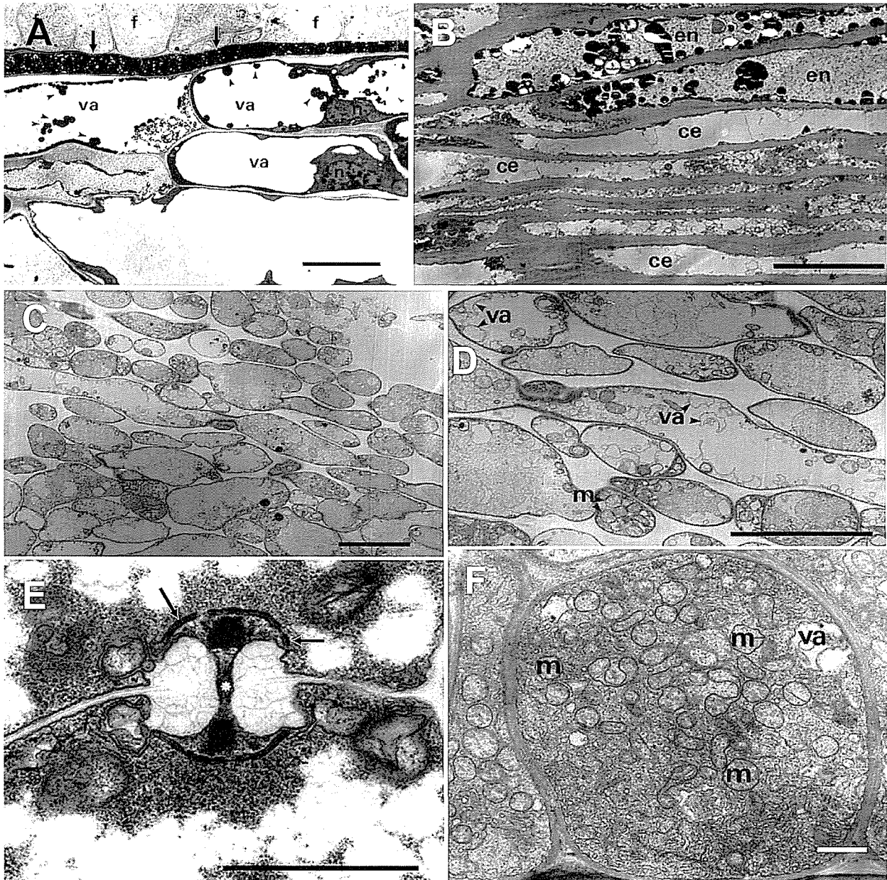
図－ 6. 菌根各部の超薄切片像 (1)
