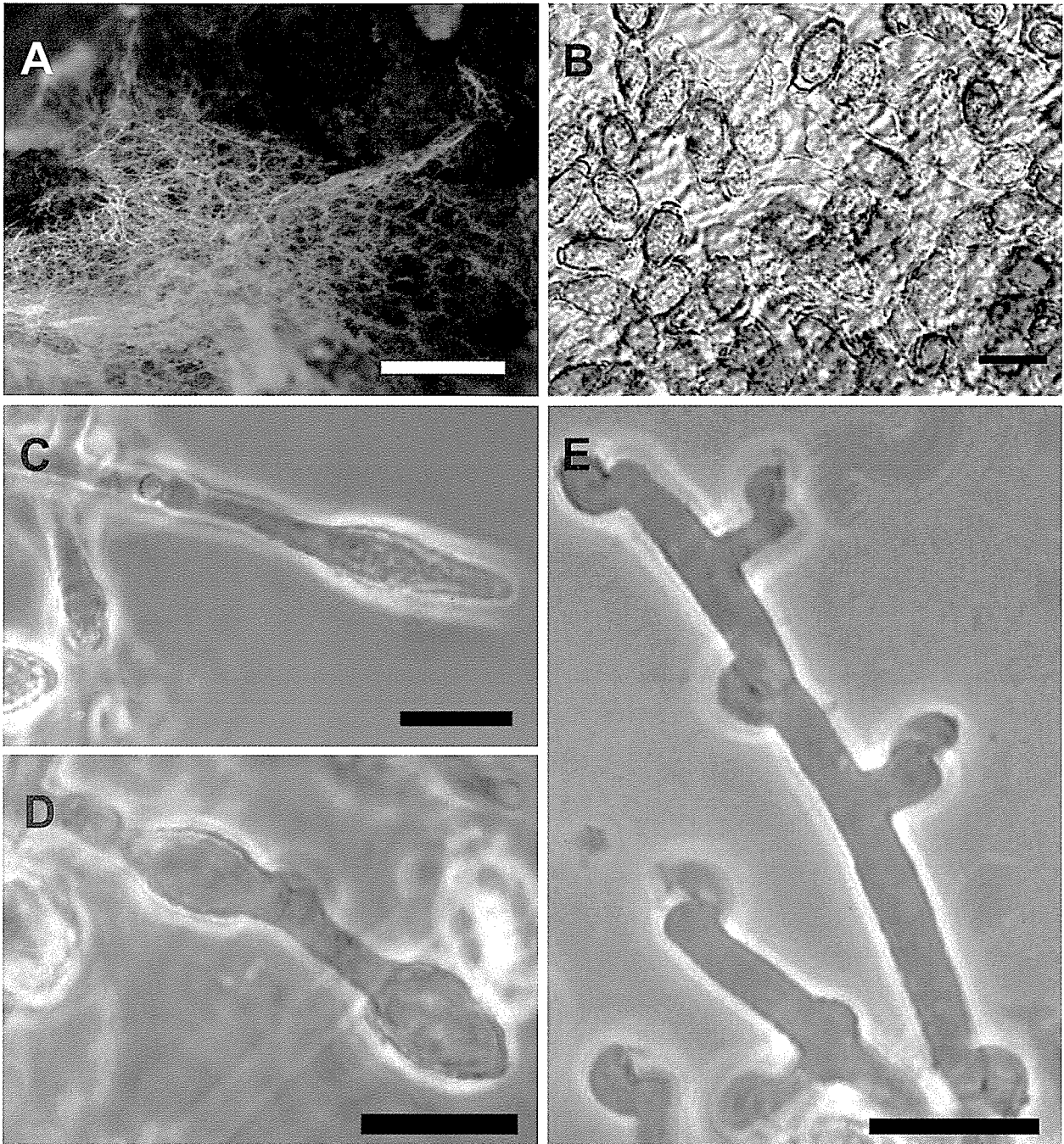
図－ 2. Entoloma clypeatum f. hybridum の厚壁孢子
