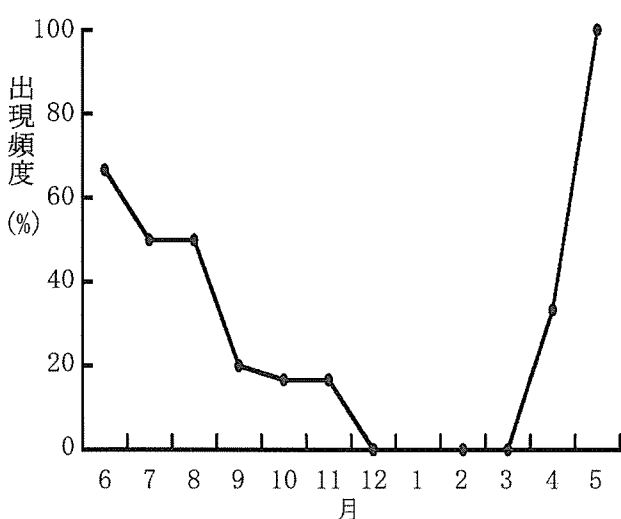
図－9. Entoloma saepium がウメの根に形成する菌根の月毎の出現頻度
