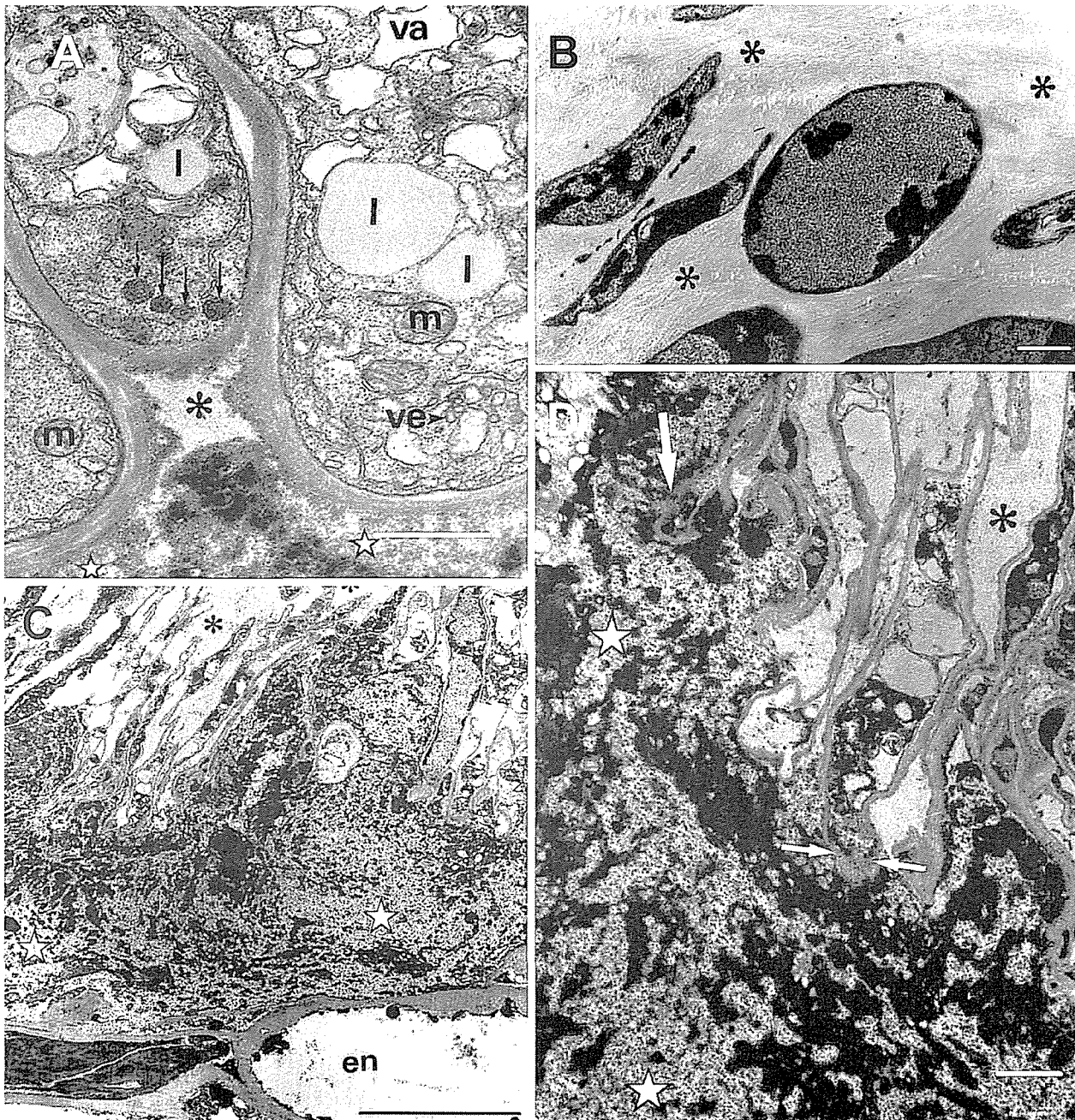
図－ 8．菌根各部の超薄切片像 (3)
