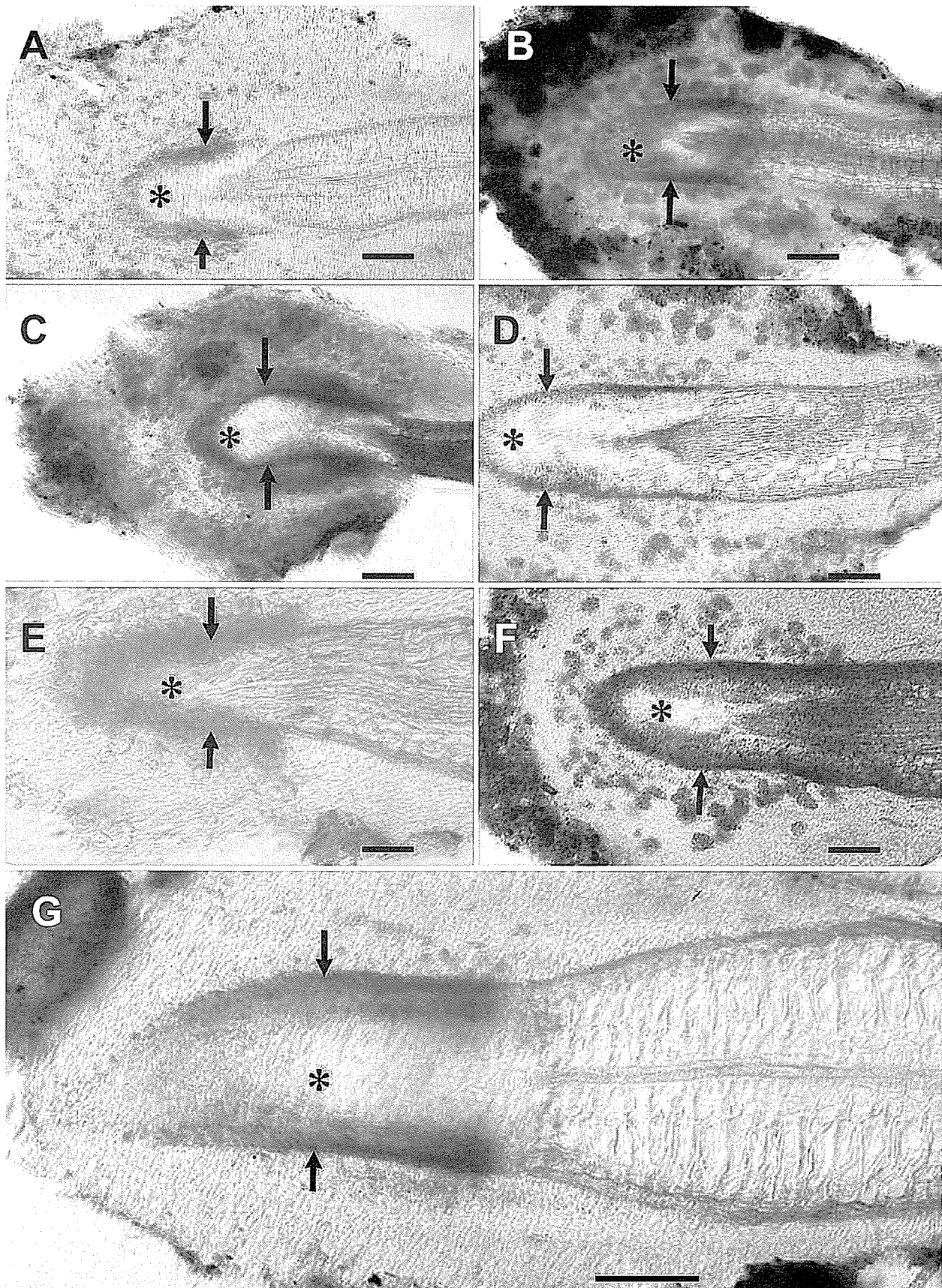
図ー 5. 様々な植物樹下で観察されたハルシメジ類の菌根の縦断切片
