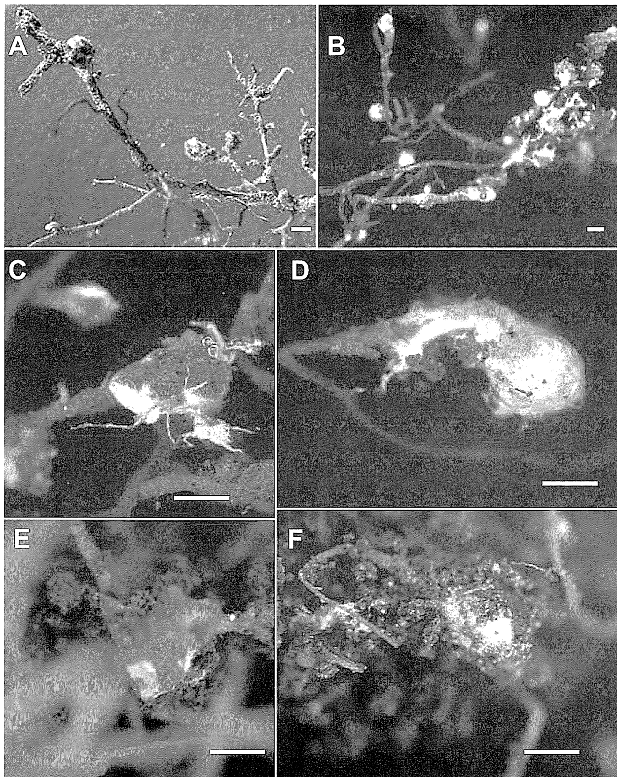
図－ 4. 様々な植物樹下で観察されたハルシメジ類の菌根
