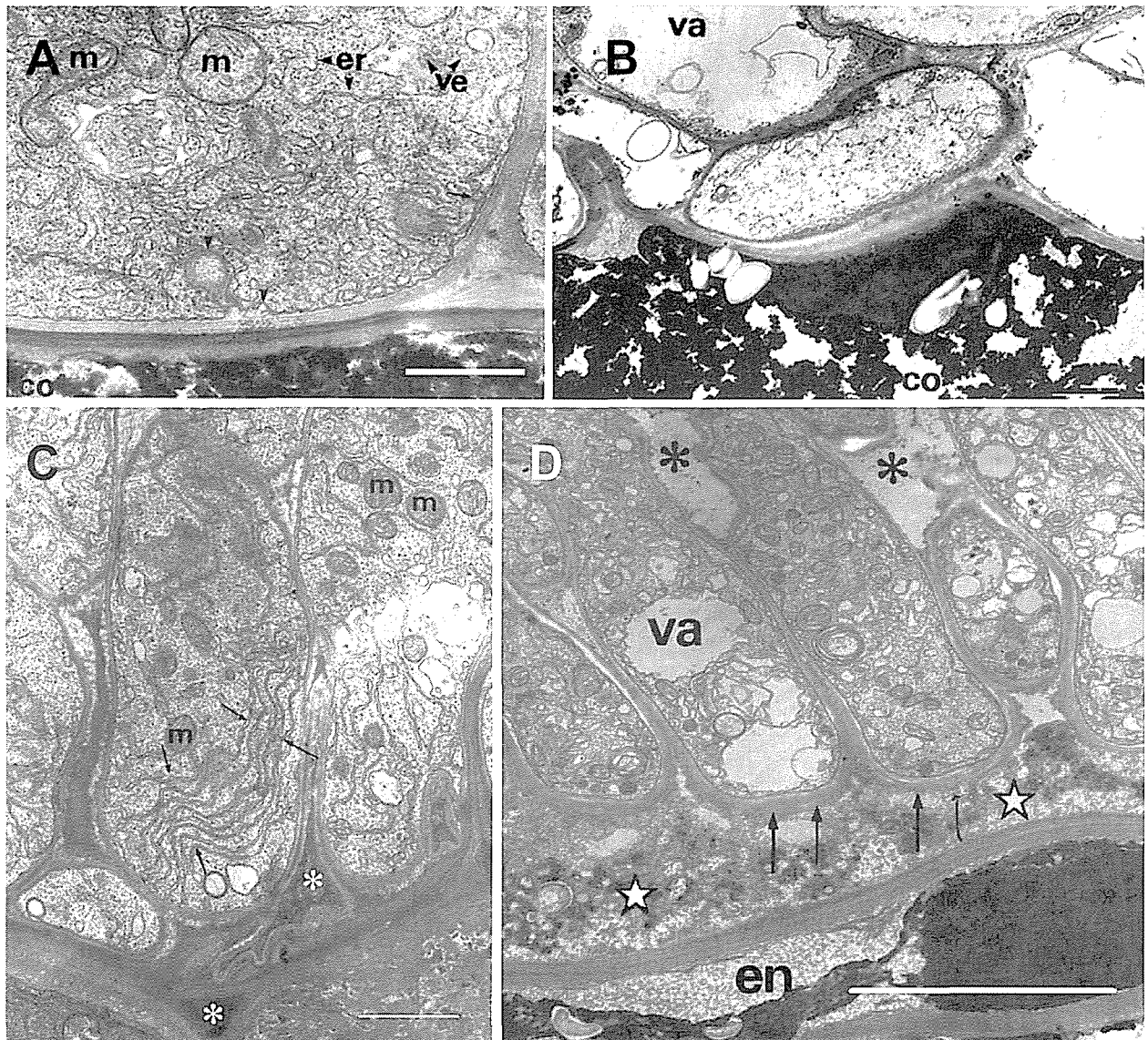
図一 7. 菌根各部の超薄切片像 (2)
