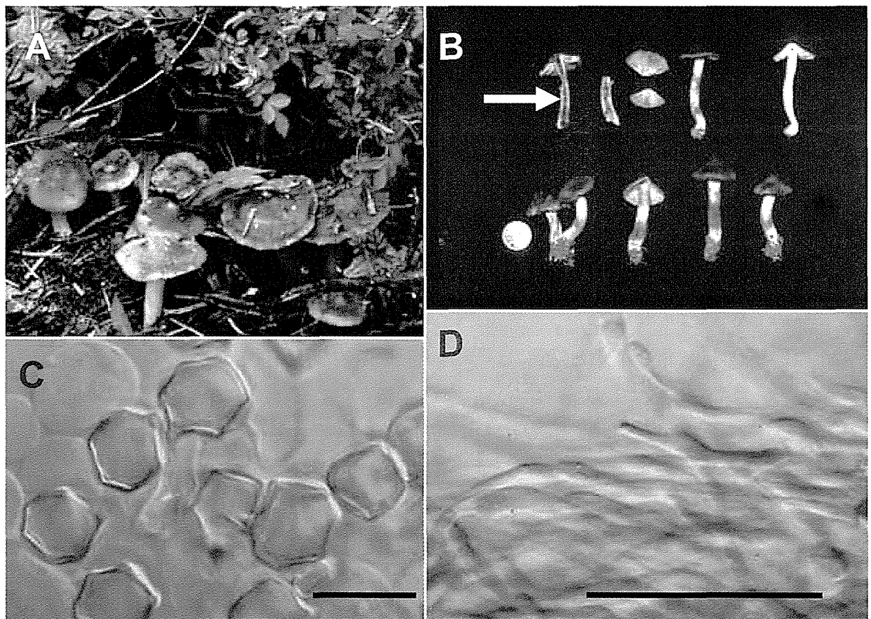
図－1. Entoloma clypeatum f. hybridum
